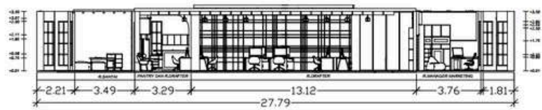
POTONGAN A-A' SKALA 1 : 150
