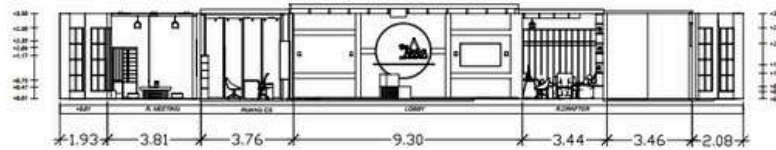
POTONGAN B-B' SKALA 1 : 150
