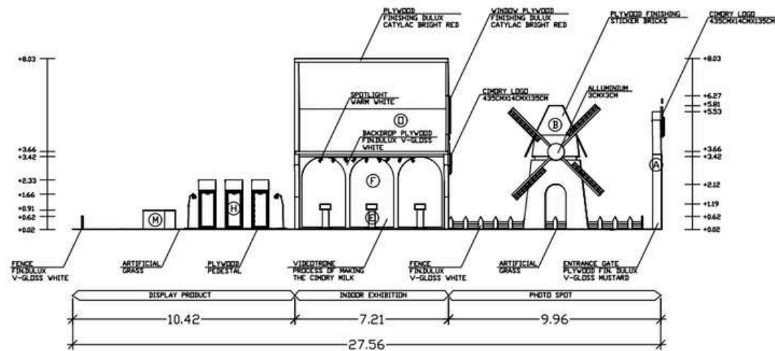
POTONGAN A-A' SKALA 1:200
