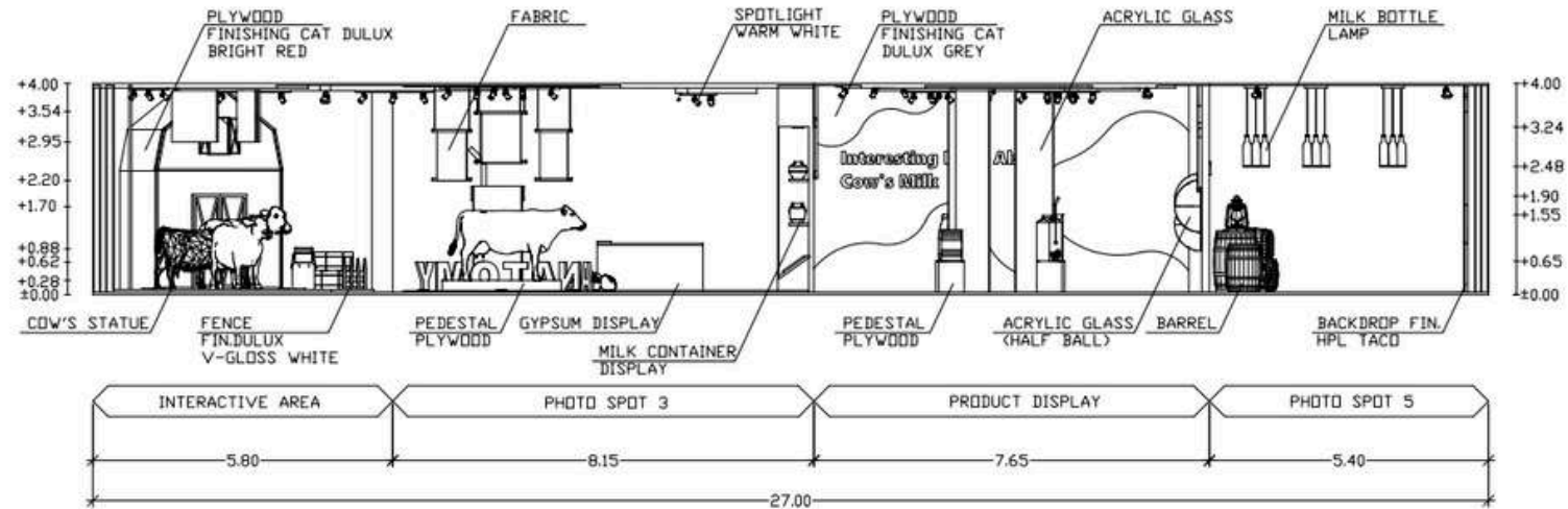
POTONGAN B-B' SKALA 1:100
