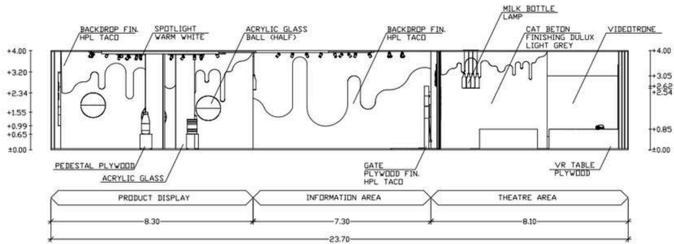
POTONGAN C-C' SKALA 1:100
