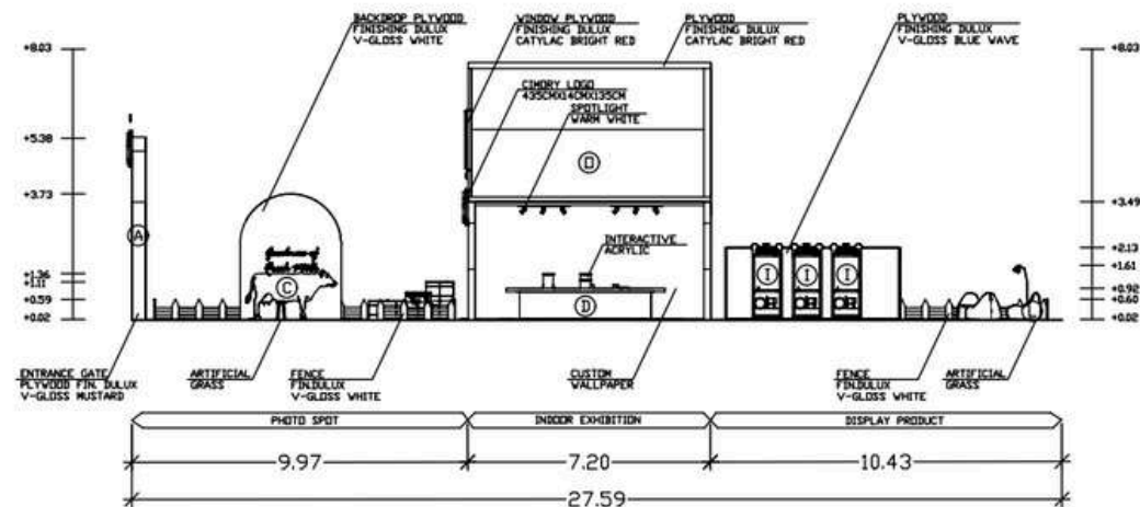
POTONGAN A-A' SKALA 1:200
