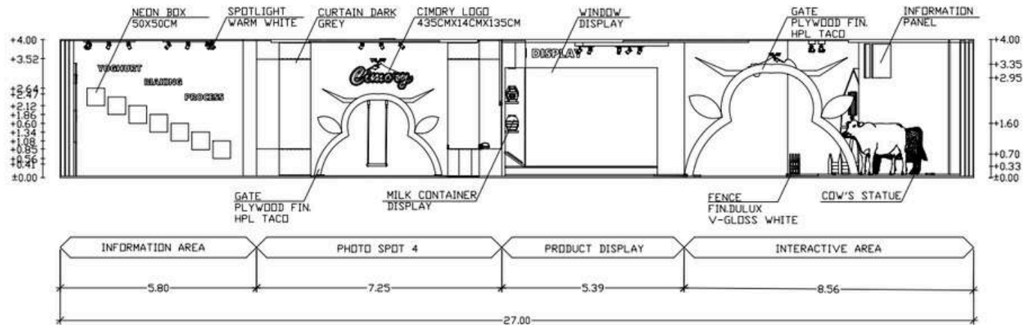
POTONGAN D-D' SKALA 1:100
