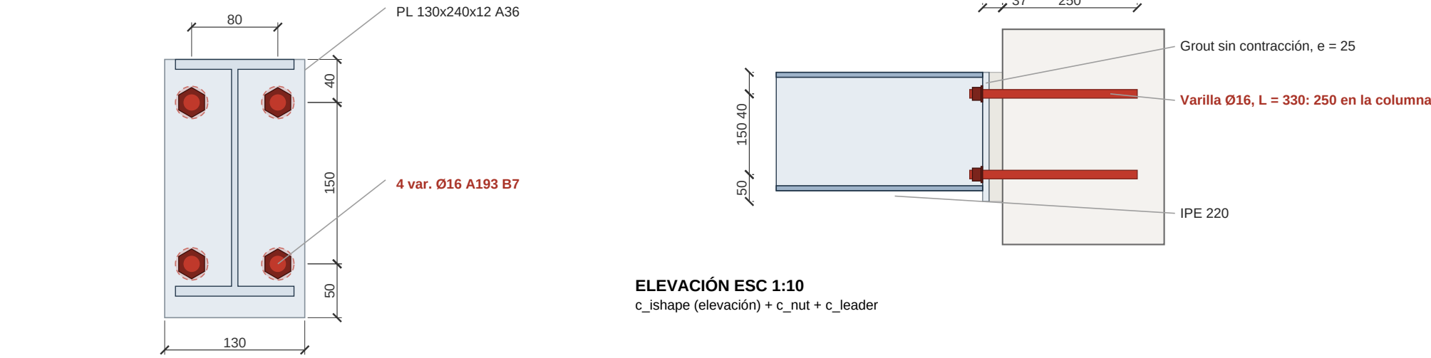
VISTA DE FRENTE ESC 1:5
