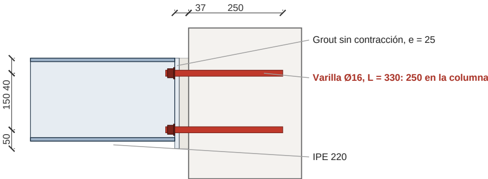
ELEVACIÓN ESC 1:10 c_ishape (elevación) + c_nut + c_leader
