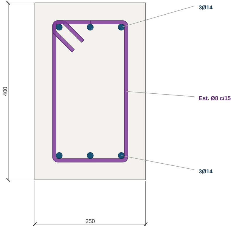
CORTE A-A: V-2 25x40 ESC 1:5 c_rc_section + c_rc_dims + c_rc_labels
