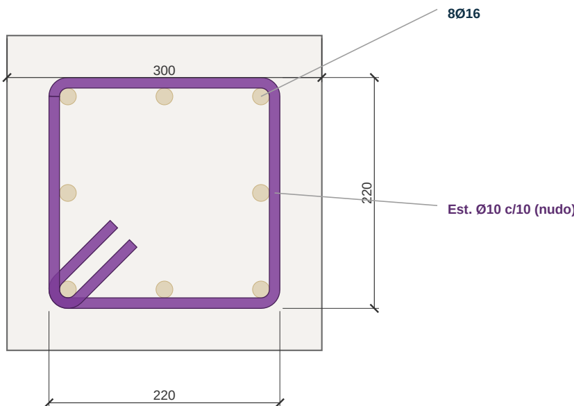
COLUMNA C 30x30 ESC 1:5 c_column_tie (cota interior: estribo) + c_rc_labels
