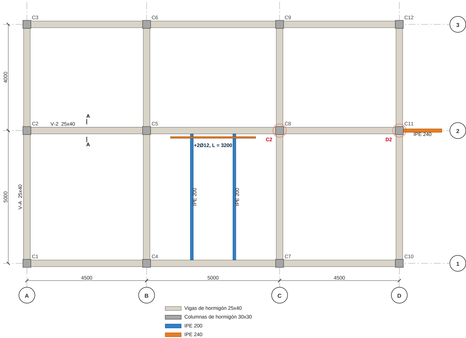
PLANTA DE UBICACIÓN ESC 1:75 c_grid, c_member, c_column_mark, c_node, c_rebar, c_cutmark, c_dim_chain, c_legend
