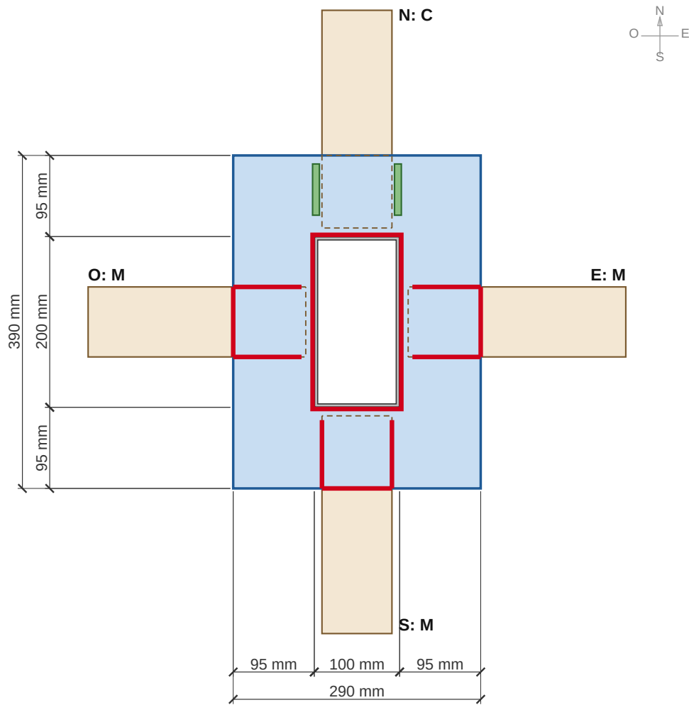
DETALLE 24 - UNIÓN D3, COLLARÍN TIPO A O N E S: M C M M. Lado de 200 mm de la columna en dirección N-S.
