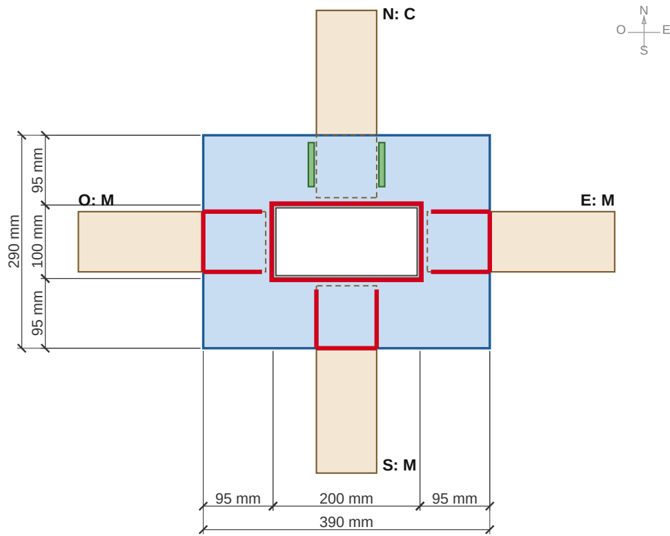
DETALLE 20 - UNIÓN C3, COLLARÍN TIPO A O N E S: M C M M. Lado de 200 mm de la columna en dirección E-O.
