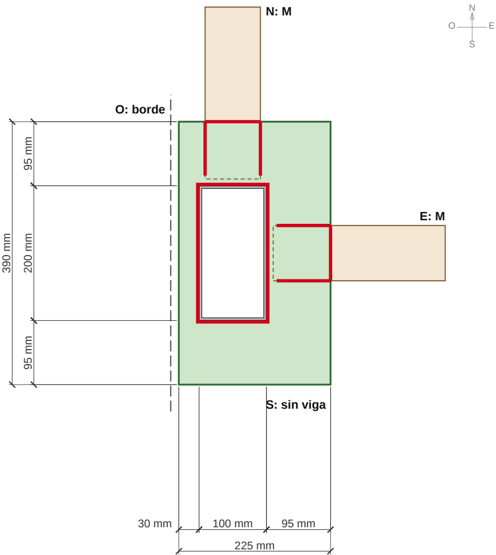
DETALLE 13 - UNIÓN A4, COLLARÍN TIPO B O N E S: — M M —. Lado de 200 mm de la columna en dirección N-S.
