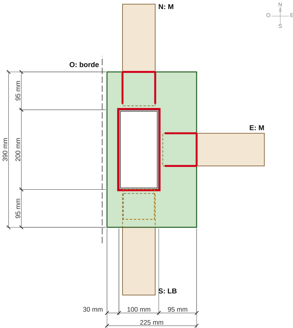
DETALLE 11 - UNIÓN A2, COLLARÍN TIPO B O N E S: — M M LB. Lado de 200 mm de la columna en dirección N-S.
