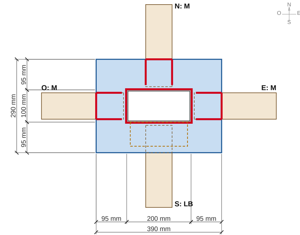
DETALLE 19 - UNIÓN C2, COLLARÍN TIPO A O N E S: M M M LB. Lado de 200 mm de la columna en dirección E-O.
