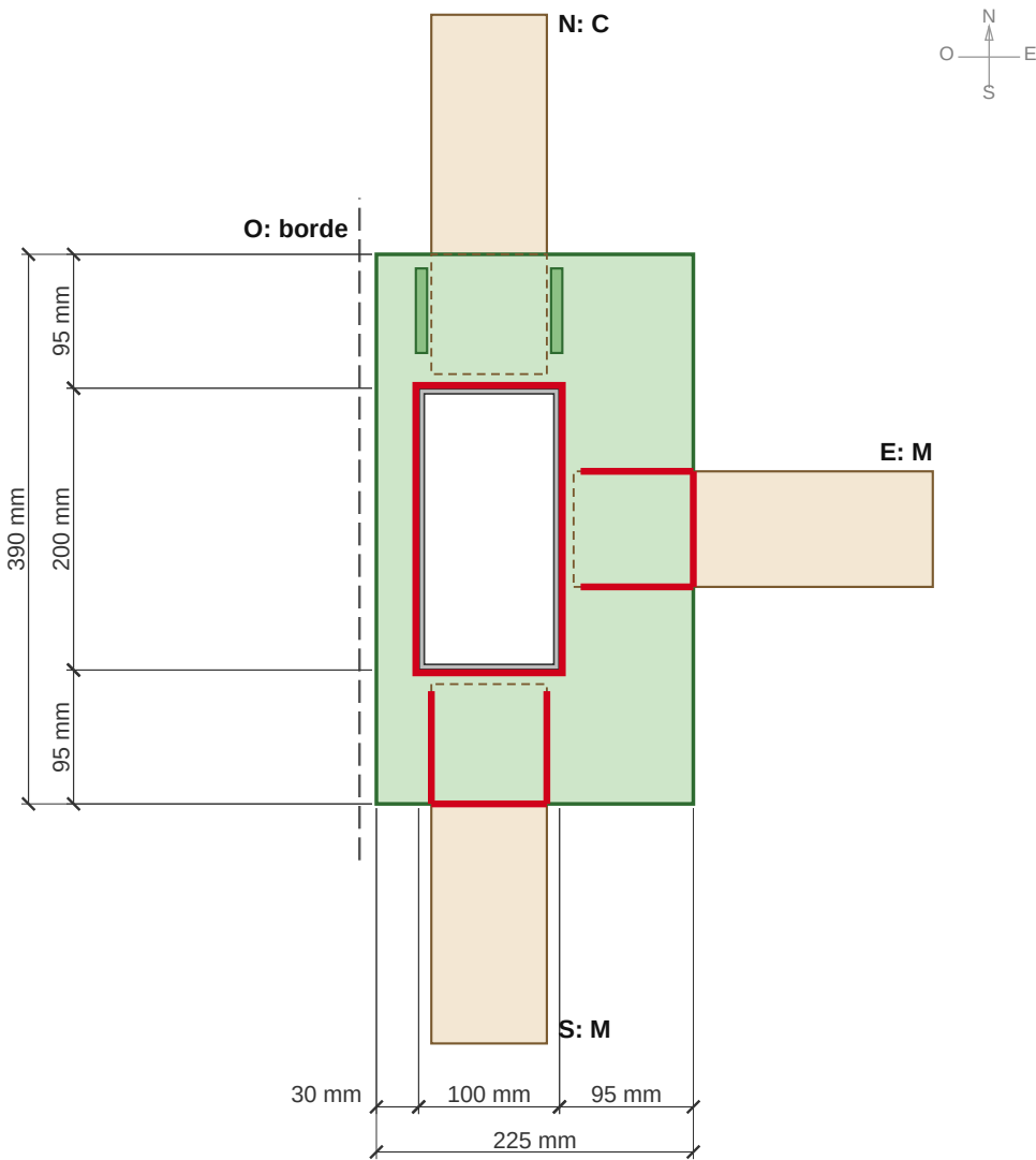
DETALLE 12 - UNIÓN A3, COLLARÍN TIPO B O N E S: — C M M. Lado de 200 mm de la columna en dirección N-S.
