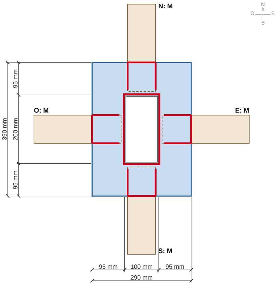
DETALLE 22 - UNIÓN D1, COLLARÍN TIPO A O N E S: M M M M. Lado de 200 mm de la columna en dirección N-S.
