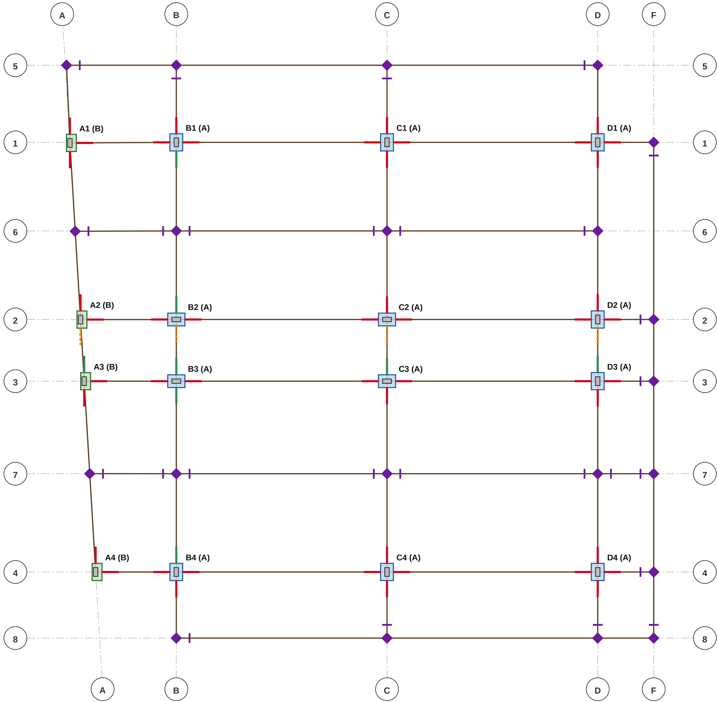
DETALLE 1 - PLANTA GENERAL DE UNIONES Collarines coloreados por tipo. Las correas no se muestran.
