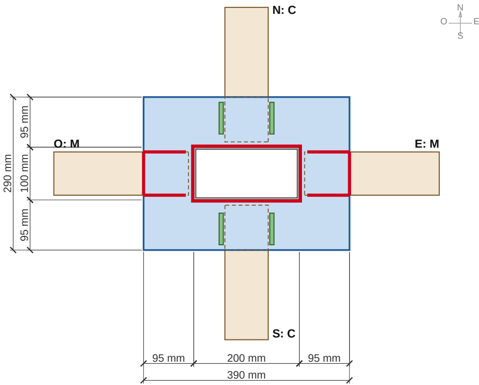
DETALLE 16 - UNIÓN B3, COLLARÍN TIPO A O N E S: M C M C. Lado de 200 mm de la columna en dirección E-O.
