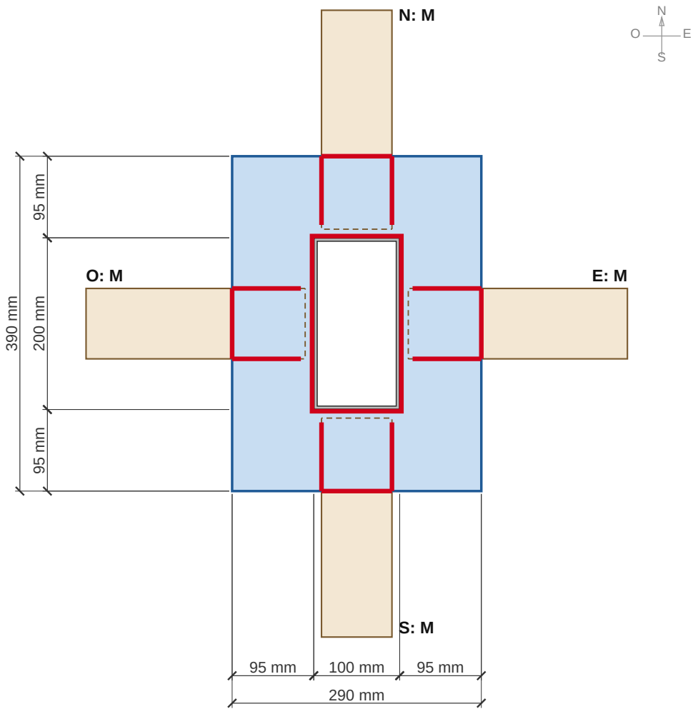
DETALLE 21 - UNIÓN C4, COLLARÍN TIPO A O N E S: M M M M. Lado de 200 mm de la columna en dirección N-S.
