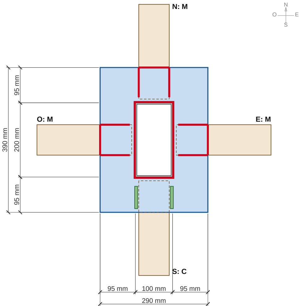
DETALLE 14 - UNIÓN B1, COLLARÍN TIPO A O N E S: M M M C. Lado de 200 mm de la columna en dirección N-S.
