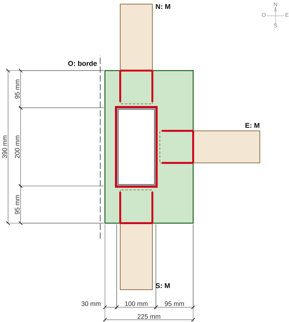
DETALLE 10 - UNIÓN A1, COLLARÍN TIPO B O N E S: — M M M. Lado de 200 mm de la columna en dirección N-S.
