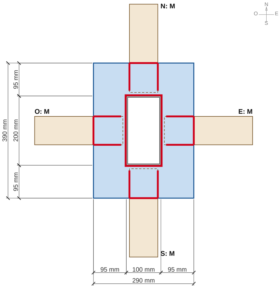
DETALLE 25 - UNIÓN D4, COLLARÍN TIPO A O N E S: M M M M. Lado de 200 mm de la columna en dirección N-S.
