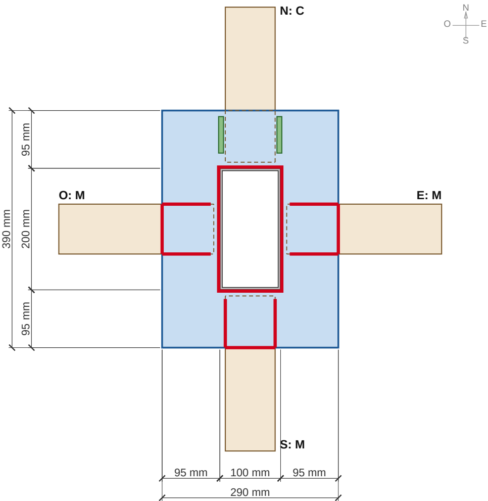
DETALLE 17 - UNIÓN B4, COLLARÍN TIPO A O N E S: M C M M. Lado de 200 mm de la columna en dirección N-S.
