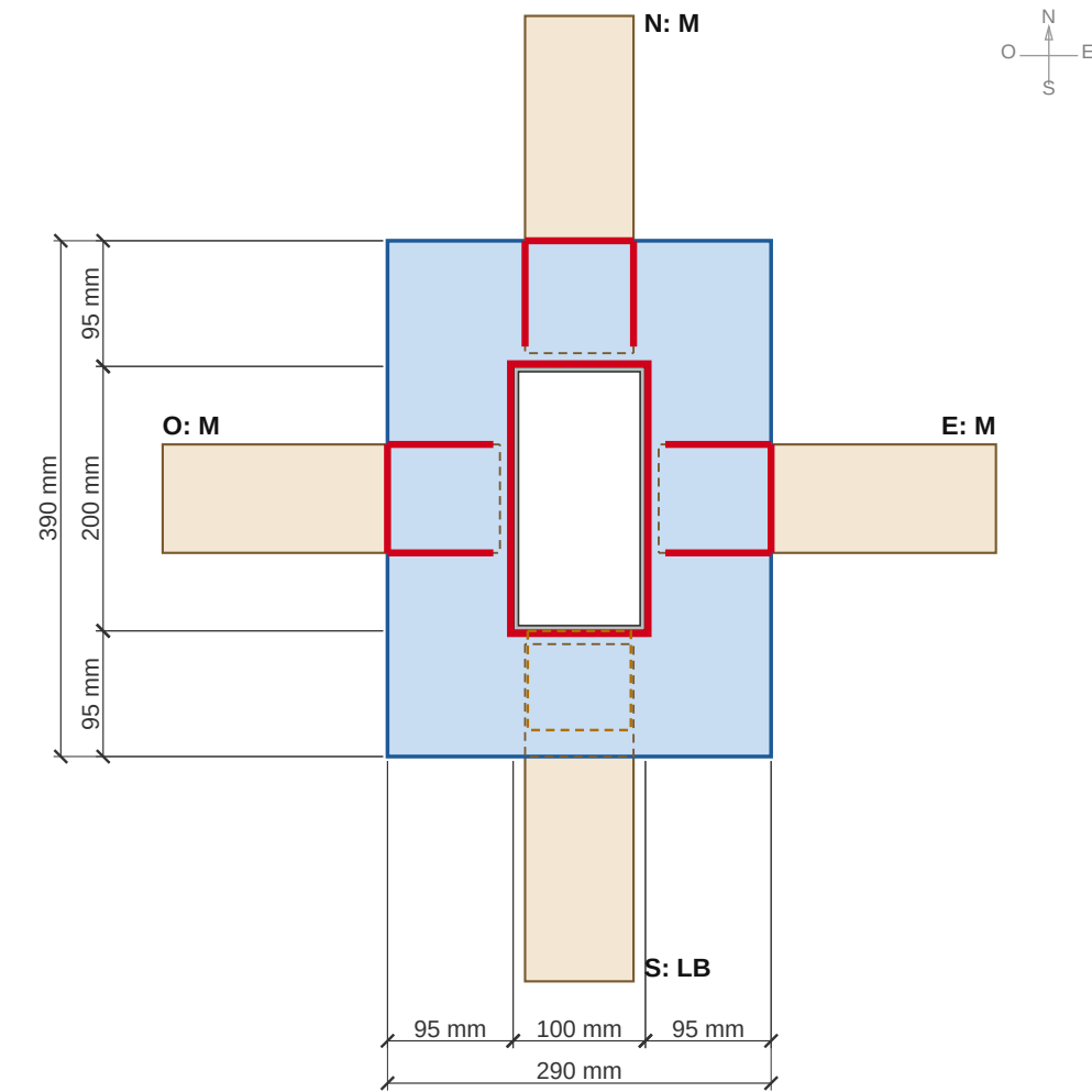
DETALLE 23 - UNIÓN D2, COLLARÍN TIPO A O N E S: M M M LB. Lado de 200 mm de la columna en dirección N-S.
