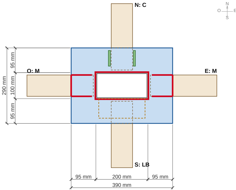
DETALLE 15 - UNIÓN B2, COLLARÍN TIPO A O N E S: M C M LB. Lado de 200 mm de la columna en dirección E-O.
