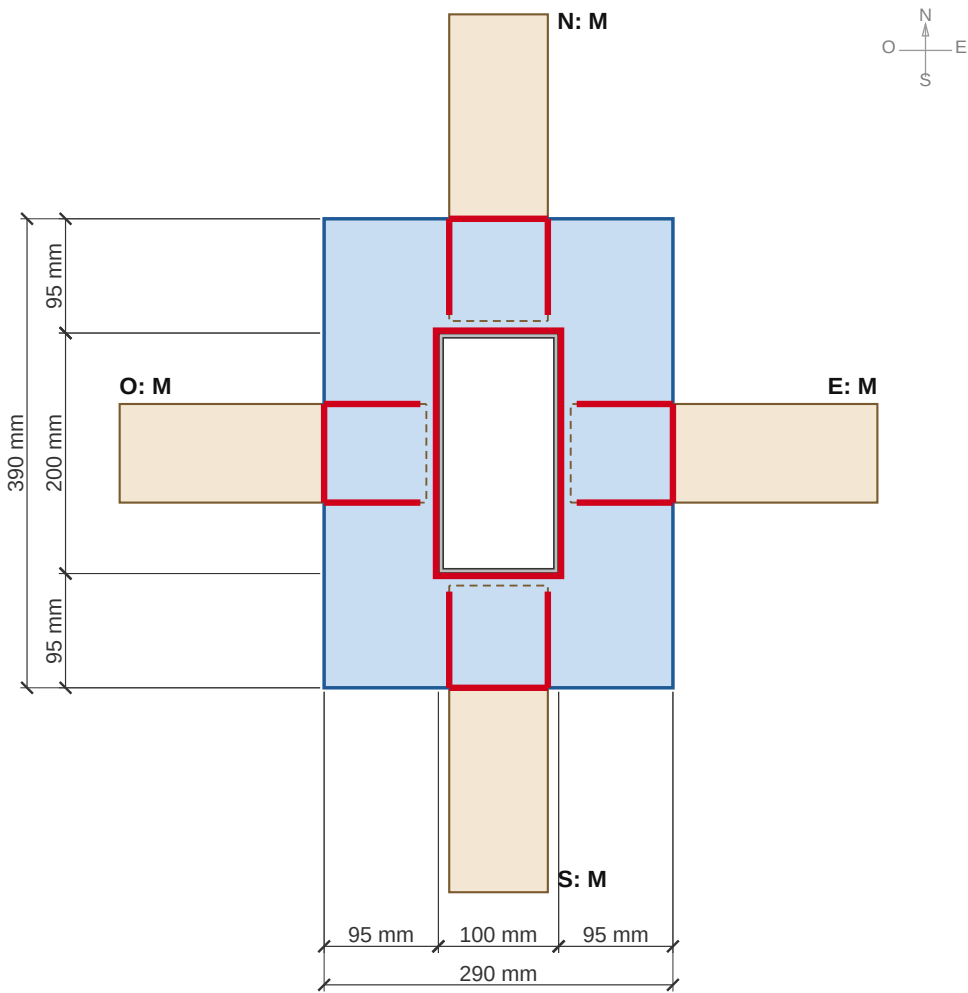
DETALLE 18 - UNIÓN C1, COLLARÍN TIPO A O N E S: M M M M. Lado de 200 mm de la columna en dirección N-S.
