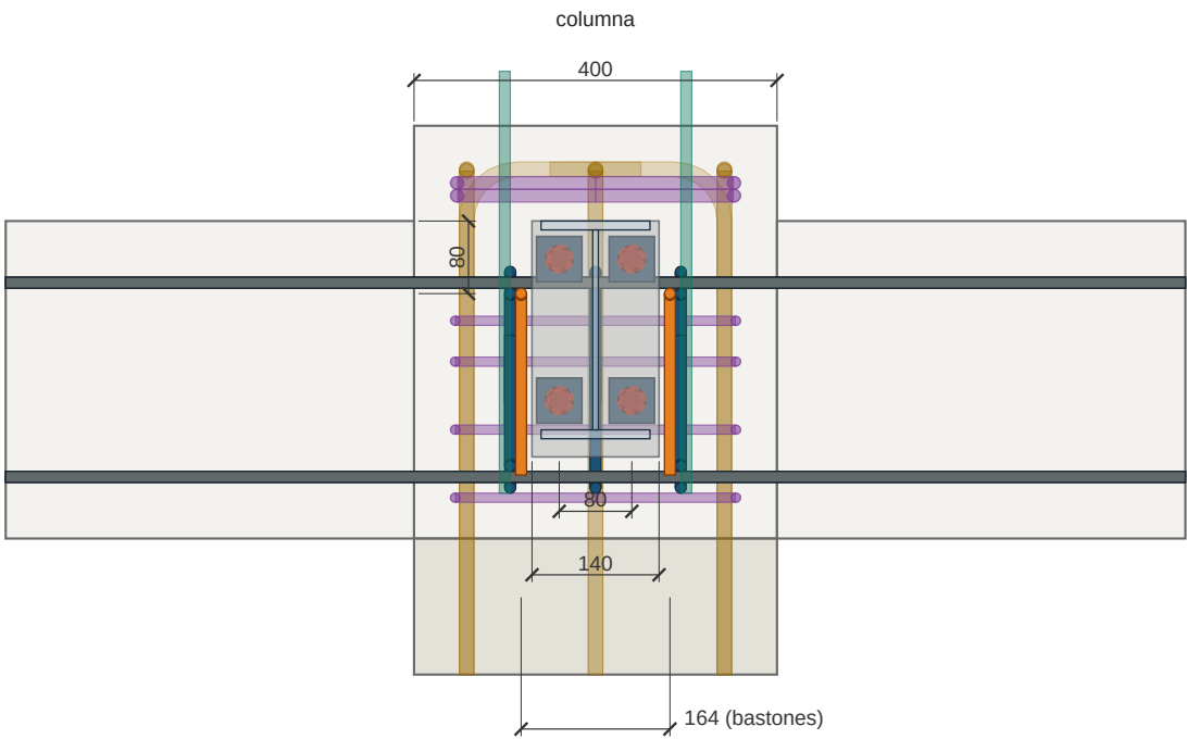
VISTA DESDE LA VIGA Sin la viga de atrás.
