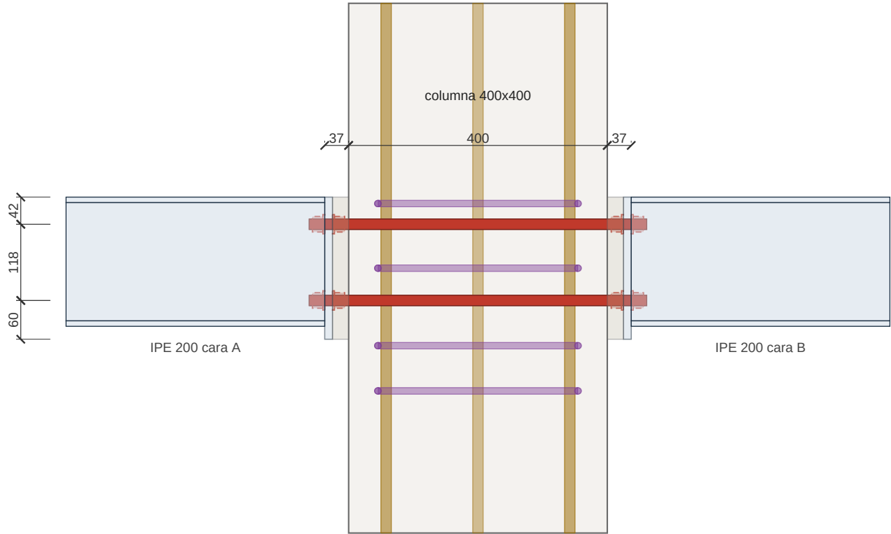
CORTE POR EL EJE DE LAS VIGAS Hormigón cortado en x = 0.
