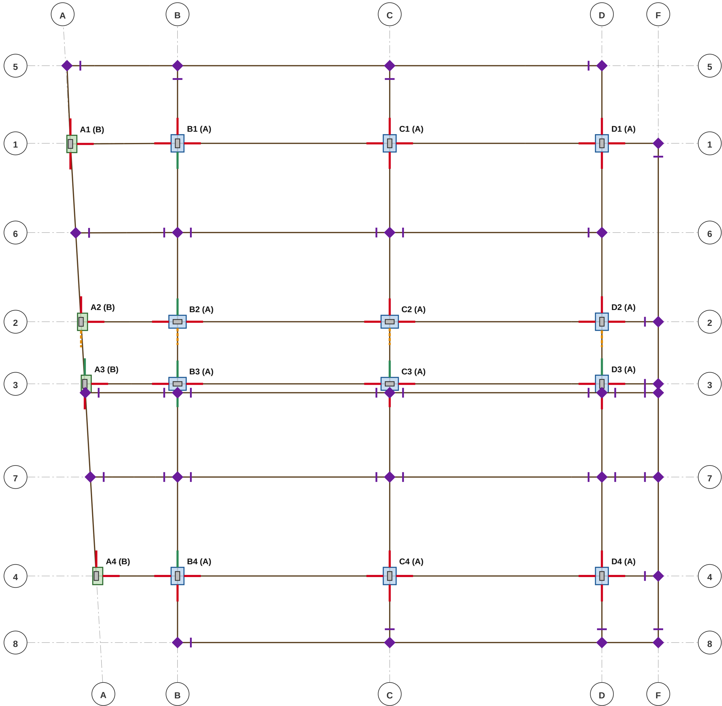
DETALLE 1 - ESQUEMA GENERAL DE UNIONES Collarines coloreados por tipo. Las correas no se muestran. Vigas a 20 cm al sur del eje 3: a nivel inferior, bajo los collarines; no interfieren con ellos.
