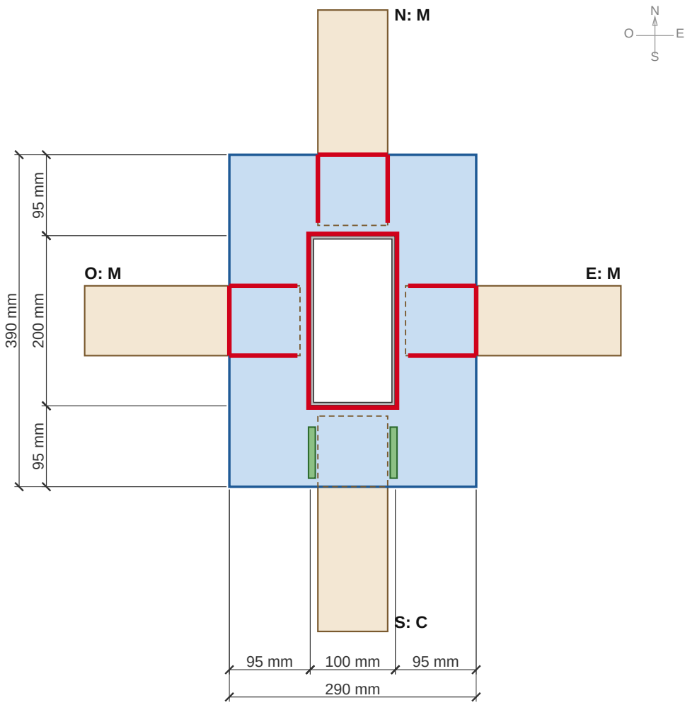
DETALLE 14 - UNIÓN B1, COLLARÍN TIPO A O N E S: M M M C. Lado de 200 mm de la columna en dirección N-S.
