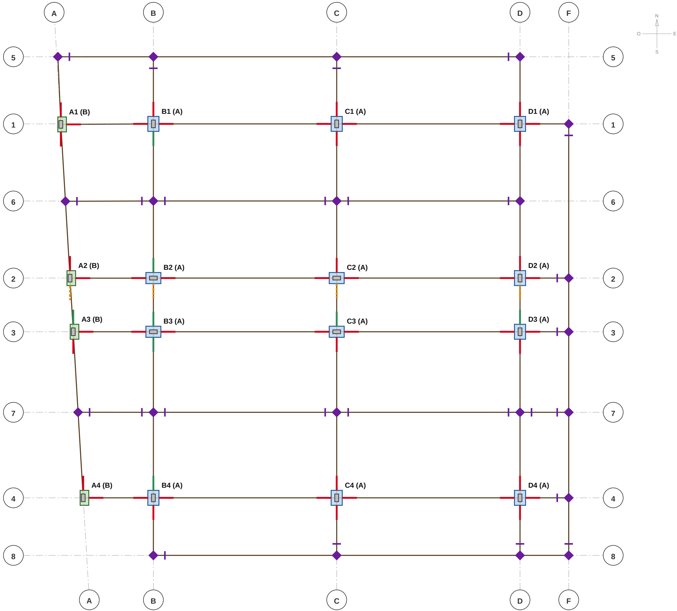
DETALLE 1 - PLANTA GENERAL DE UNIONES Collarines coloreados por tipo. Las correas no se muestran.
