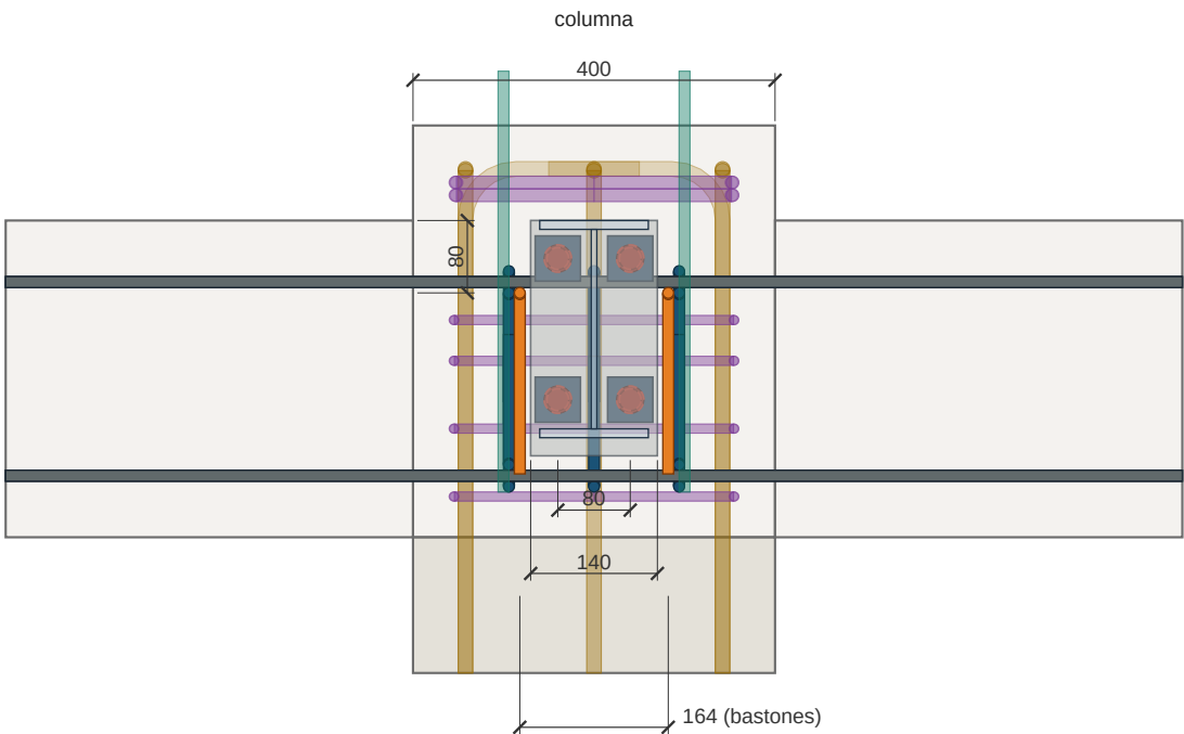
VISTA DESDE LA VIGA Sin la viga de atrás.
