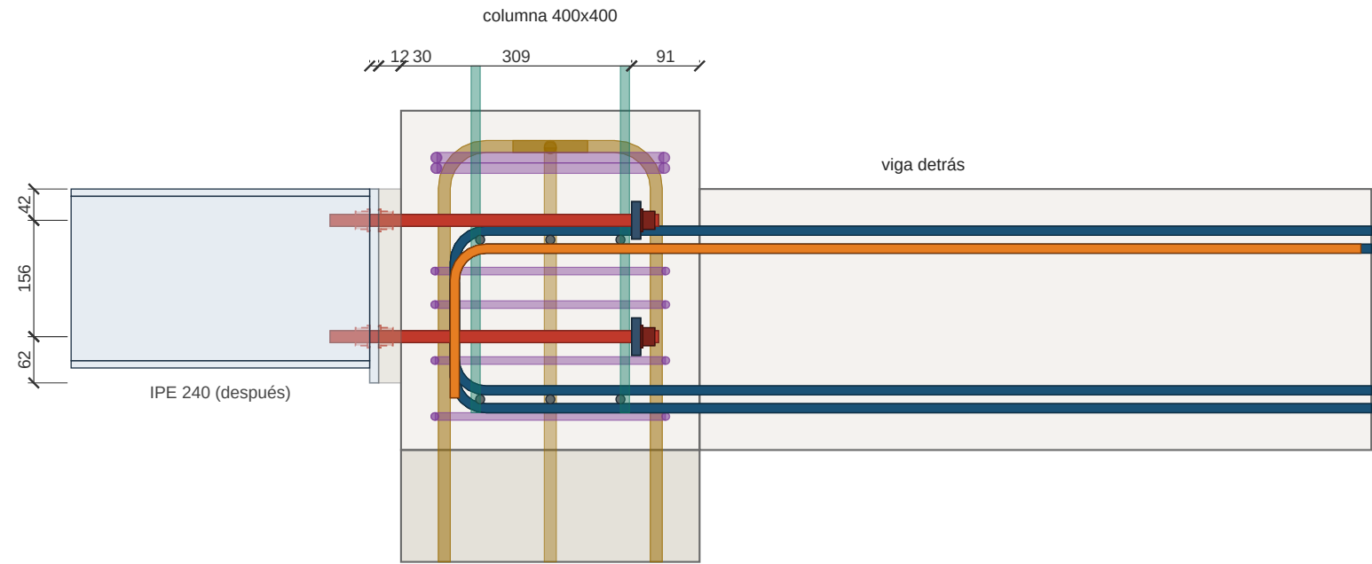
CORTE POR EL EJE DE LA VIGA Hormigón cortado en x = 0; barras y acero vistos.
