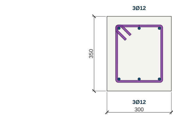
c_rc_section + c_rc_dims Sección de hormigón 30x35.
