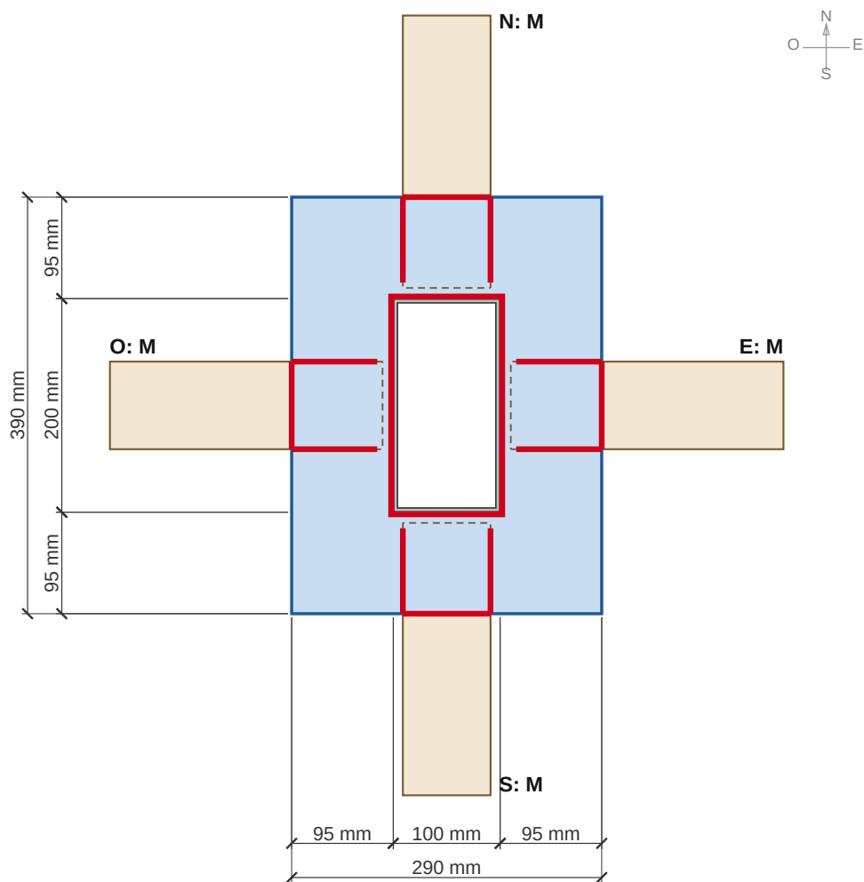
DETALLE 22 - UNIÓN D1, COLLARÍN TIPO A O N E S: M M M M. Lado de 200 mm de la columna en dirección N-S.
