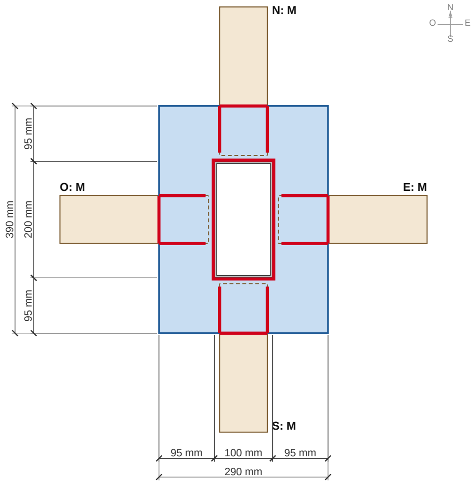
DETALLE 18 - UNIÓN C1, COLLARÍN TIPO A O N E S: M M M M. Lado de 200 mm de la columna en dirección N-S.
