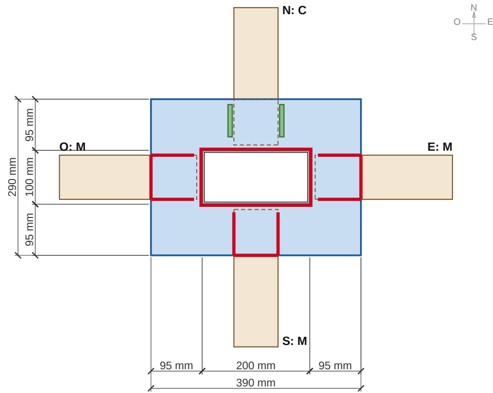
DETALLE 20 - UNIÓN C3, COLLARÍN TIPO A O N E S: M C M M. Lado de 200 mm de la columna en dirección E-O.
