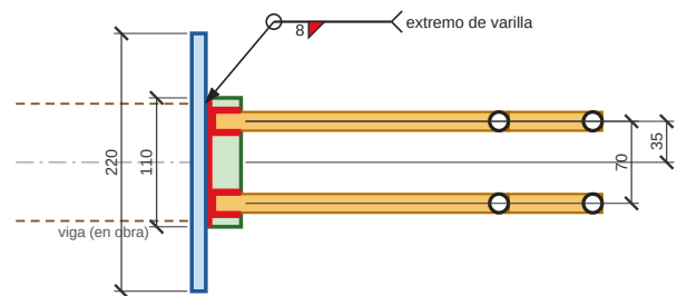
DETALLE 1.4 - TIPO E, VISTA DESDE ABAJO Vista sin la platina inferior. Abajo: varillas V1.
