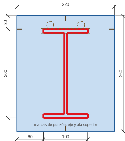
DETALLE 3.2 - TIPO C2, VISTA DE LA PLACA Vista desde afuera. En discontinuo: platina y varillas, detrás de la placa. En rojo: soldadura de obra.
