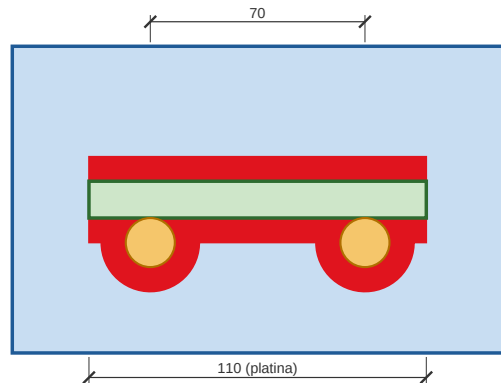
DETALLE 2.5 - SOLDADURAS DE LAS VARILLAS (AMPLIADO) Izquierda: vista lateral. Derecha: vista contra la placa, con todas las varillas. La cara cortada de la varilla apoya en la placa; no se suelda. El cordón de 8 mm sigue la platina y rodea cada varilla. Donde la varilla toca la platina no hay soldadura.
