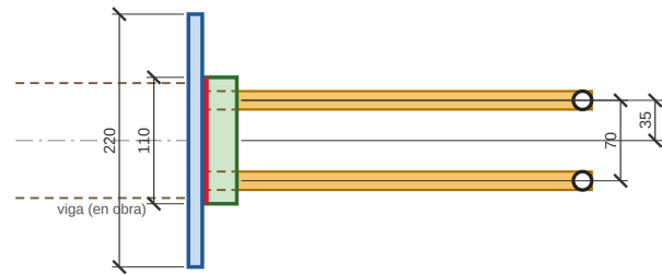
DETALLE 3.4 - TIPO C2, VISTA DESDE ABAJO Vista sin la platina inferior. Varillas encima, en discontinuo.
