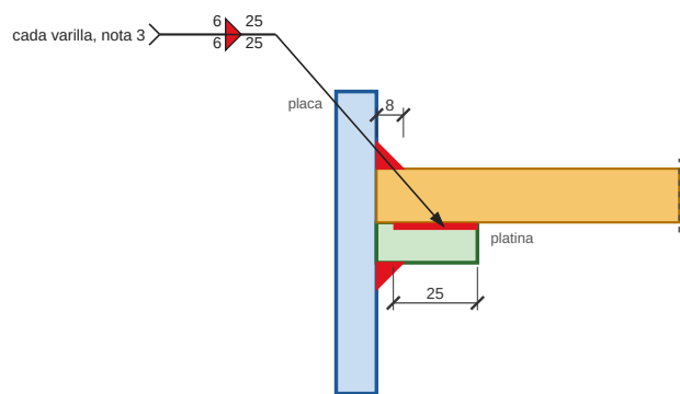
DETALLE 3.3 - TIPO C2, VISTA DESDE ARRIBA Varillas sobre la platina.
