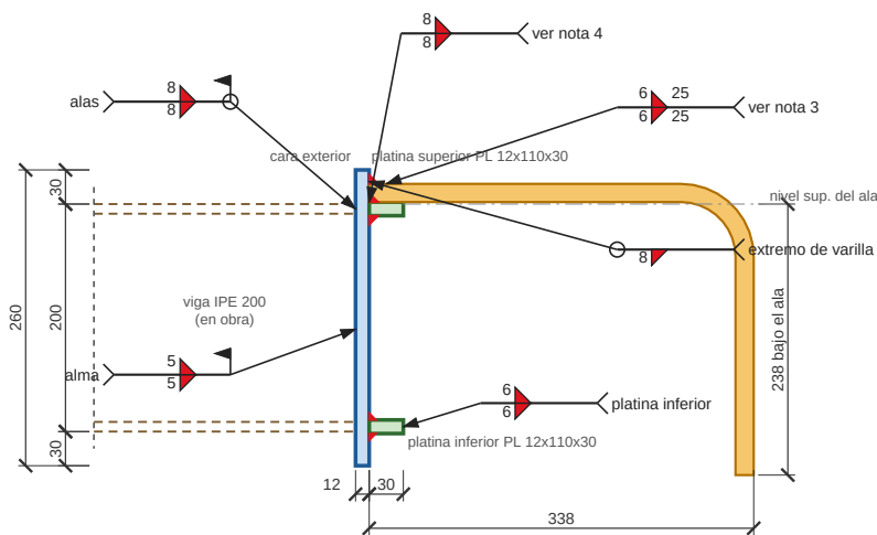
DETALLE 3.1 - TIPO C2, ELEVACIÓN LATERAL Viga en discontinuo: se suelda en obra. Cotas desde la cara exterior de la placa.
