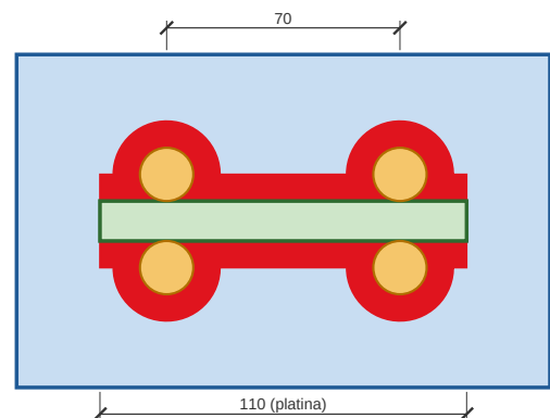
DETALLE 1.5 - SOLDADURAS DE LAS VARILLAS (AMPLIADO) Izquierda: vista lateral. Derecha: vista contra la placa, con todas las varillas. La cara cortada de la varilla apoya en la placa; no se suelda. El cordón de 8 mm sigue la platina y rodea cada varilla. Donde la varilla toca la platina no hay soldadura.
