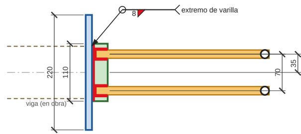
DETALLE 2.4 - TIPO C1, VISTA DESDE ABAJO Vista sin la platina inferior. Varillas bajo la platina.
