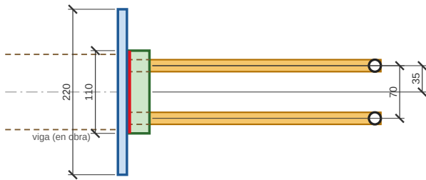
DETALLE 2.3 - TIPO C1, VISTA DESDE ARRIBA Varillas debajo de la platina, en discontinuo.
