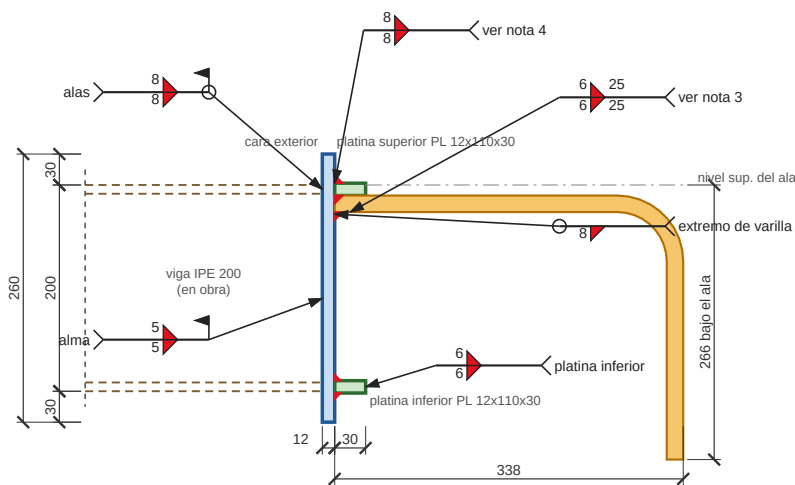
DETALLE 2.1 - TIPO C1, ELEVACIÓN LATERAL Viga en discontinuo: se suelda en obra. Cotas desde la cara exterior de la placa.
