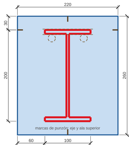
DETALLE 2.2 - TIPO C1, VISTA DE LA PLACA Vista desde afuera. En discontinuo: platina y varillas, detrás de la placa. En rojo: soldadura de obra.
