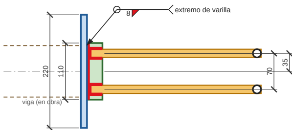
DETALLE 3.3 - TIPO C2, VISTA DESDE ARRIBA Varillas sobre la platina.
