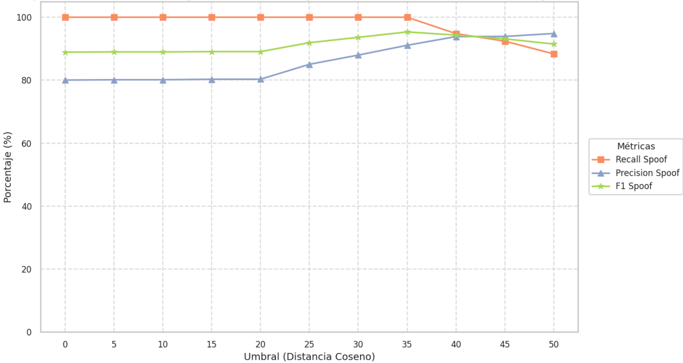
Comparación de métricas para usuarios impostores vs Umbral de Distancia ponderada
