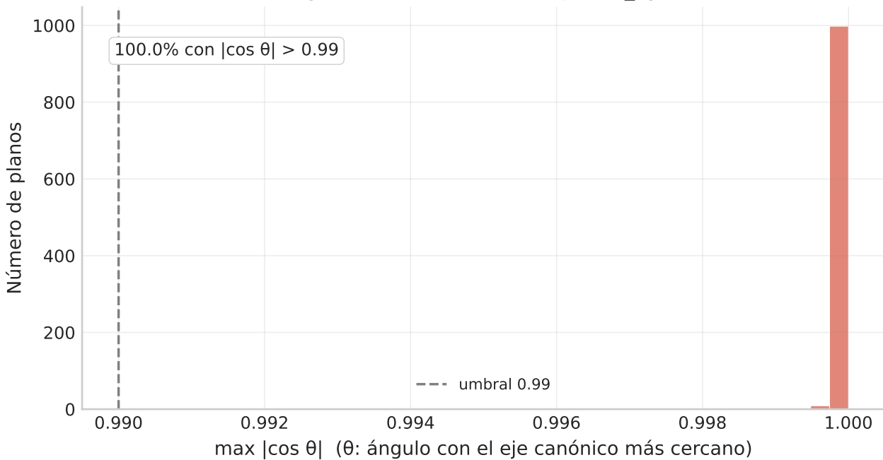
Alineación de normales de plano a ejes canónicos X/Y/Z (plane_sym)
