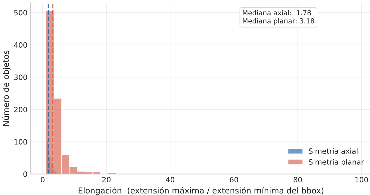
Distribución de la elongación del bounding box por objeto
