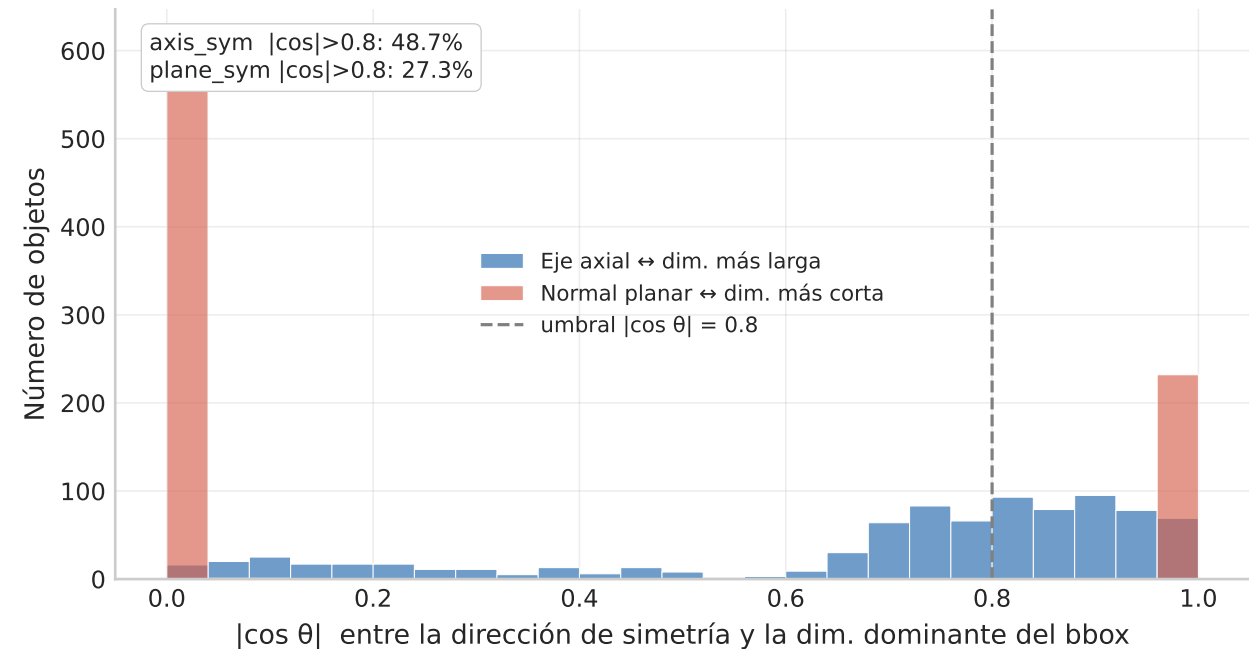
¿Se alinea la simetría con la elongación del bounding box?
