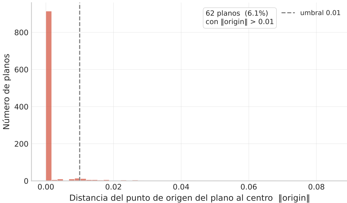
Centrado de los planos de simetría respecto al origen de coordenadas ¿Pasan los planos de simetría por el origen? (plane_sym)
