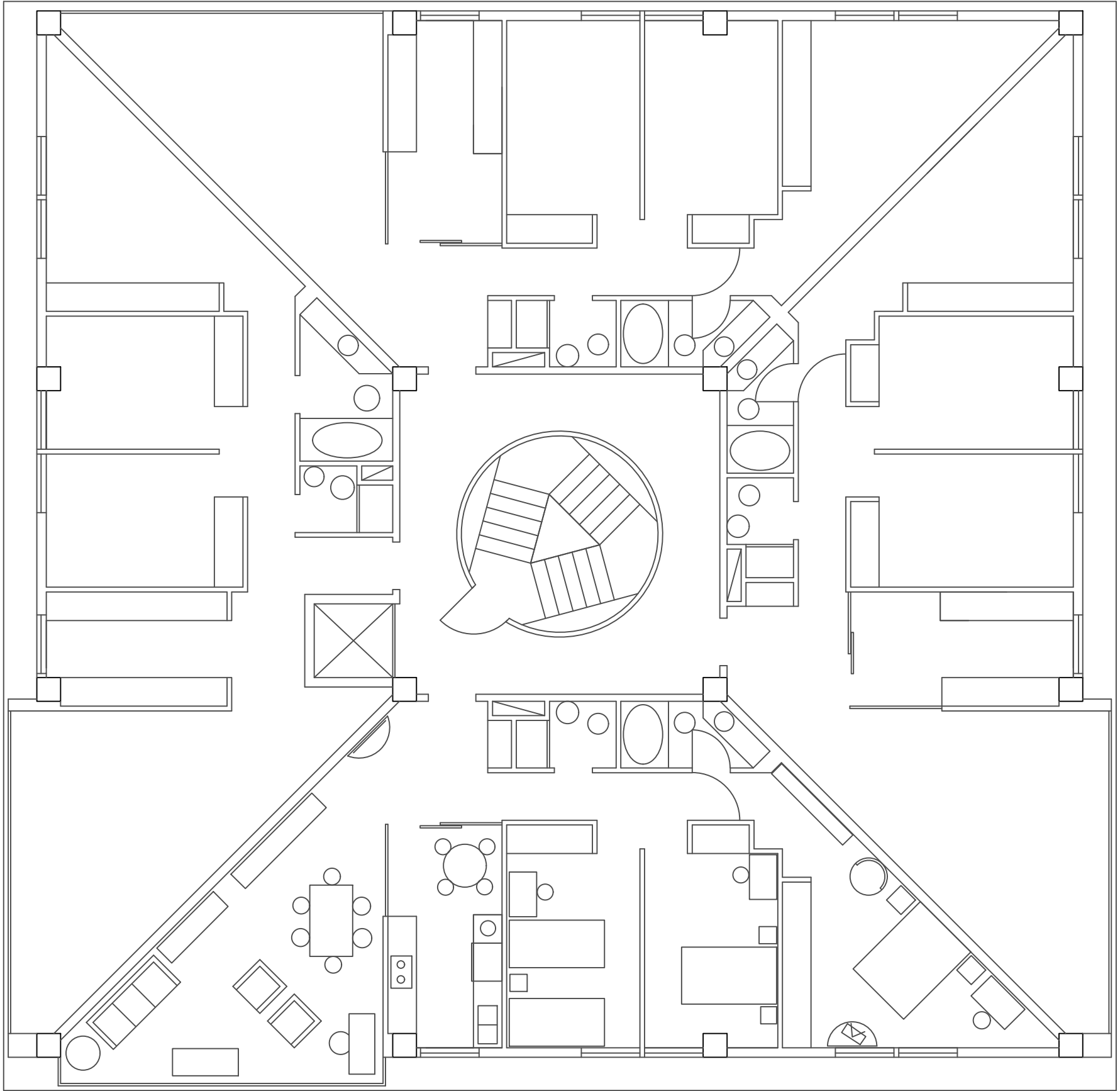
PLANTA TIPO
