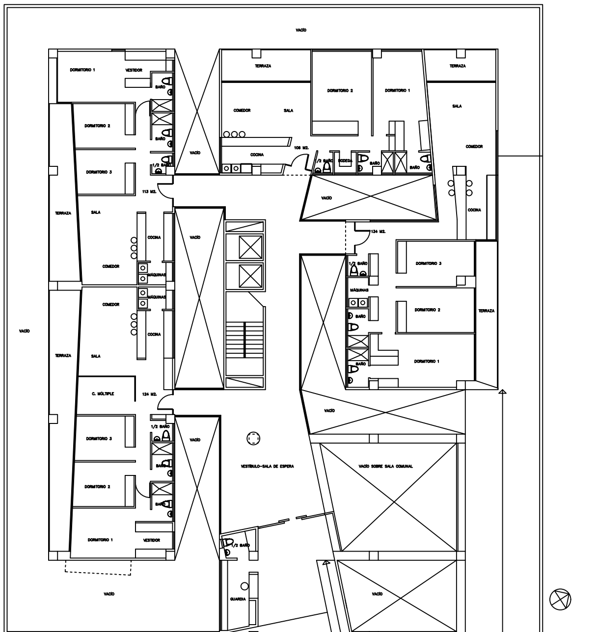
PLANTA BAJA
