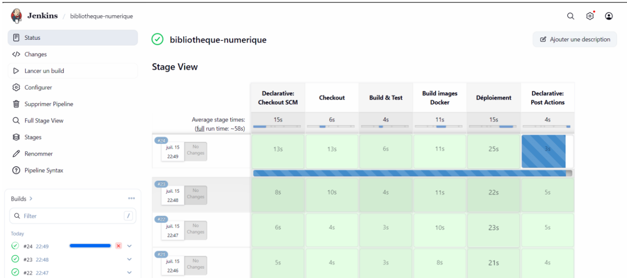
Figure — Exécution du pipeline dans Jenkins
