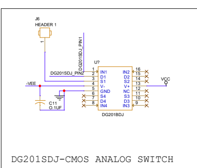
DG201SDJ-CMOS ANALOG SWITCH
