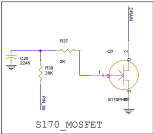
S170_MOSFET
