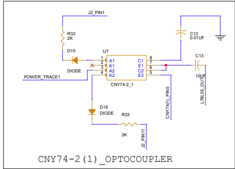
CNY74-2 (1)_OPTOCOUPLER
