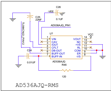
AD536AJQ-RMS
