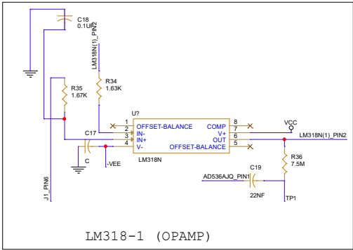
LM318-1 (OPAMP)
