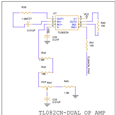
TL082CN-DUAL OP AMP
