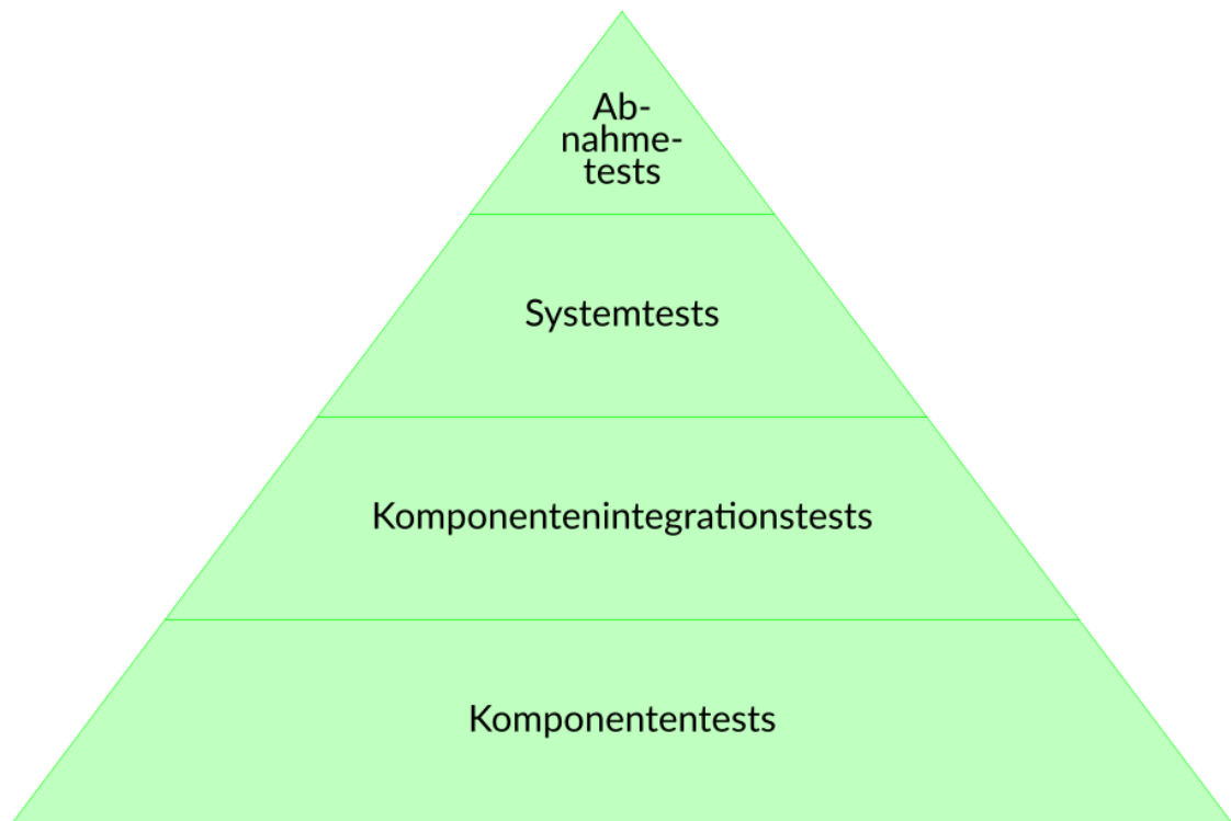
Abbildung 3: Die Testpyramide
