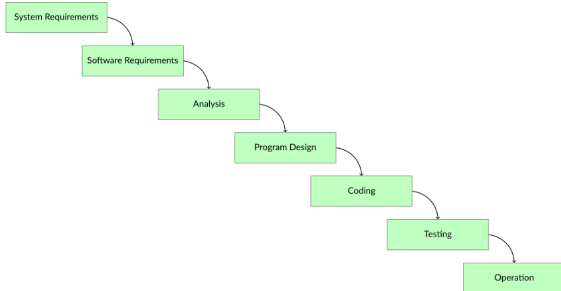
Abbildung 1: Das Wasserfallmodell
