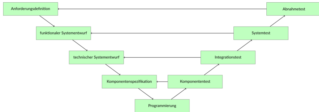
Abbildung 2: Das V-Modell
