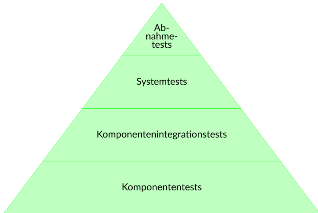
Abbildung 3: Die Testpyramide
