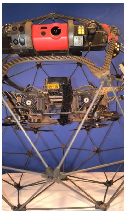
Imagem 2 – Equipamento pertencente a VALE – Mina Cauê
