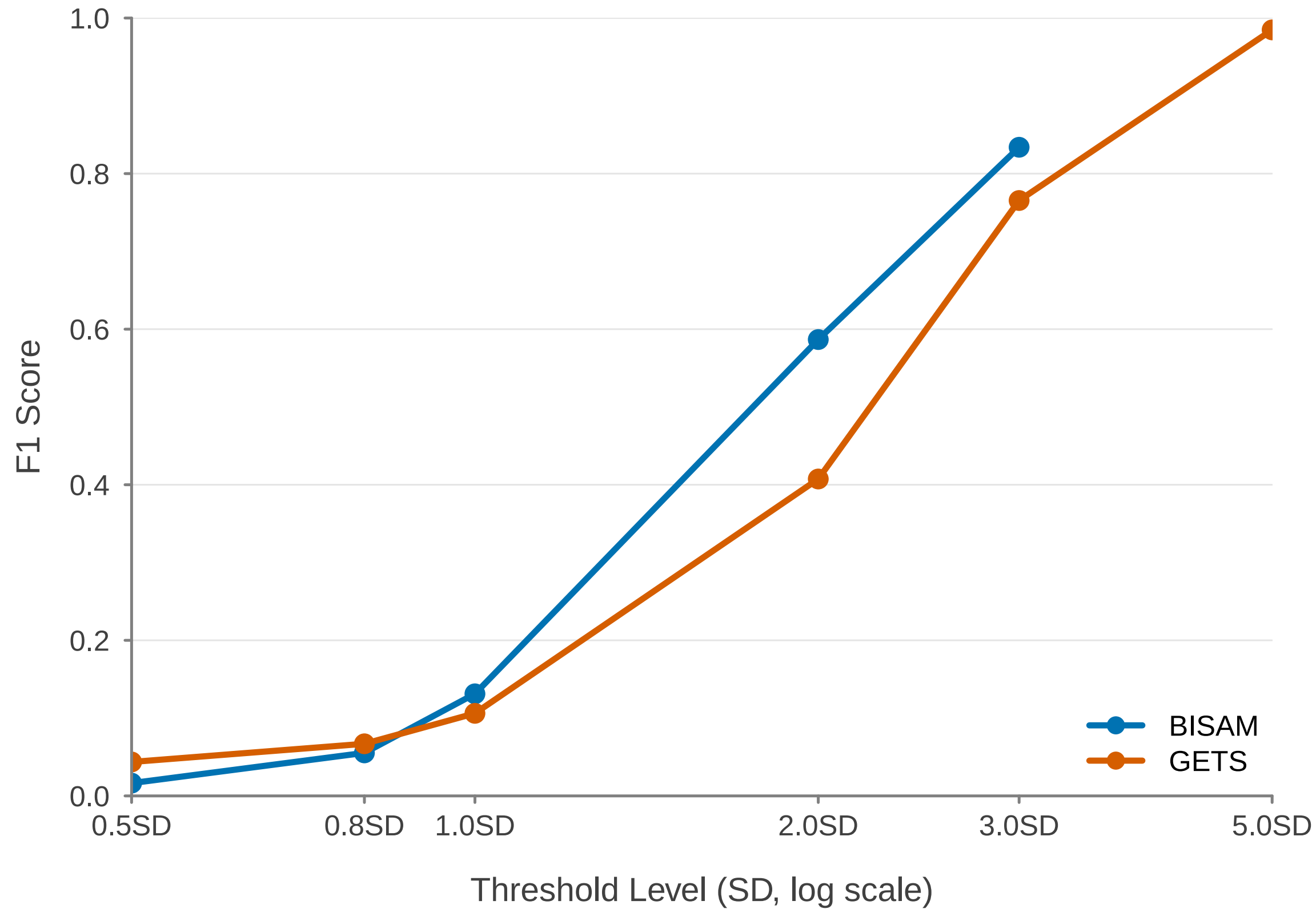
F1 Score Comparison
