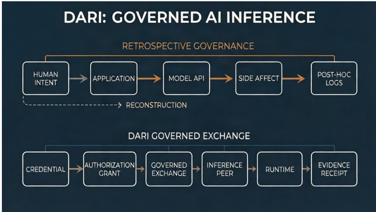
그림 1: 사후 거버넌스와 DARI의 거버넌스 적용 교환 비교. DARI는 제한적 권한, 모델 신원, 인과 증거를 실제 처리 경로의 조건으로 표현한다. 본 그림은 개념도이며 측정 데이터나 구현 범위에 관한 주장을 포함하지 않는다.
