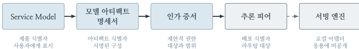
그림 3: 서버가 주도하는 모델 결정의 프로토콜 설계. 제품, 아티팩트, 배포 신원은 거버넌스 릴레이가 등록된 추론 피어를 결정할 때까지 구분된다. 서빙 엔진은 로컬 구현 요소이며 응용이 선택할 수 있는 엔드포인트가 아니다.
