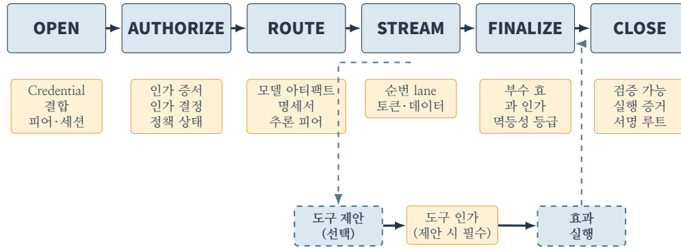
그림 2: 거버넌스 적용 교환의 프로토콜 설계도. 보호 대상 작업은 정해진 순서에 따라 권한을 검증한 뒤 진행된다. 모델이 생성한 도구 제안은 실행 전에 독립적인 인가 전이를 거쳐야 한다. 본 그림은 의도한 의미론을 설명하며 구현 범위를 측정할 결과가 아니다.
