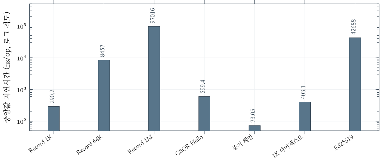
그림 4: 저장소의 TSV 데이터에서 산출한 일곱 가지 메모리 내 핵심 연산의 중량값 지연시간. 네트워크, 정책, 저장소, 모델, GPU, 토큰 생성 비용은 제외하며, 로그 척도를 사용하여 분리 측정된 CPU 비용을 식 7의 상호작용 지연 예산과 직접 비교할 수 있다.
