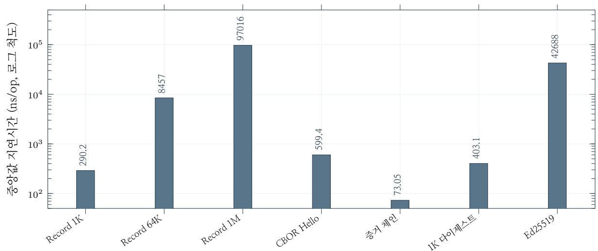
그림 4: 체크인된 TSV에서 직접 읽은 일곱 가지 메모리 내 원시 연산의 경험적 중앙값 지연시간. 로그 척도를 사용한다. 네트워크, Relay 정책, 영속화, 모델, GPU, TTFT, 토큰 생성 비용은 제외한다.
