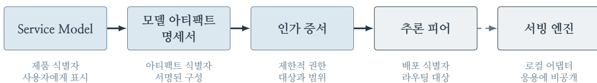
그림 3: 서버가 주도하는 모델 결정의 프로토콜 설계. 제품, 아티팩트, 배포 신원은 거버넌스 릴레이가 등록된 추론 피어를 결정할 때까지 구분된다. 서빙 엔진은 로컬 구현 요소이며 응용이 선택할 수 있는 엔드포인트가 아니다.
