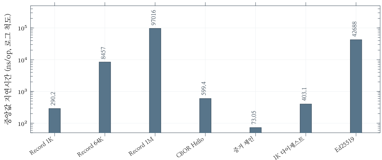
그림 4: 저장소의 TSV 데이터에서 산출한 일곱 가지 메모리 내 핵심 연산의 중앙값 지연시간. 로그 척도를 사용하였으며, 분리 측정된 CPU 비용을 식 6의 상호작용 지연 예산과 직접 비교할 수 있다.
