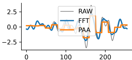
LenDB
