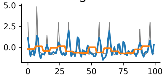
ETHZ
