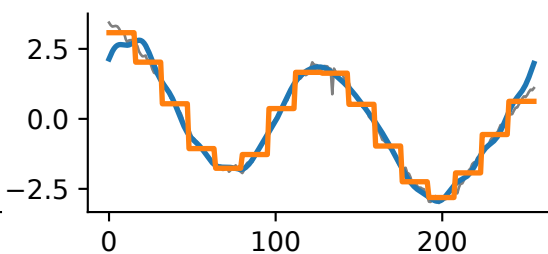
astro
