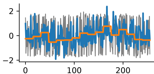
ISC-EHB-DepthPhases
