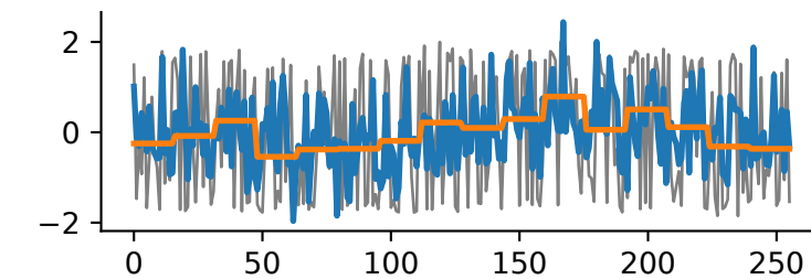
ISC-EHB-DepthPhases
