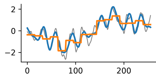
PNW
