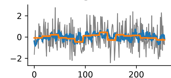
SALD
