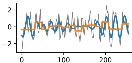
SCEDC
