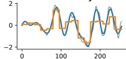
bigANN
