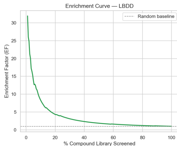
(d) PKA (MUV-548) — Enrichment curve
