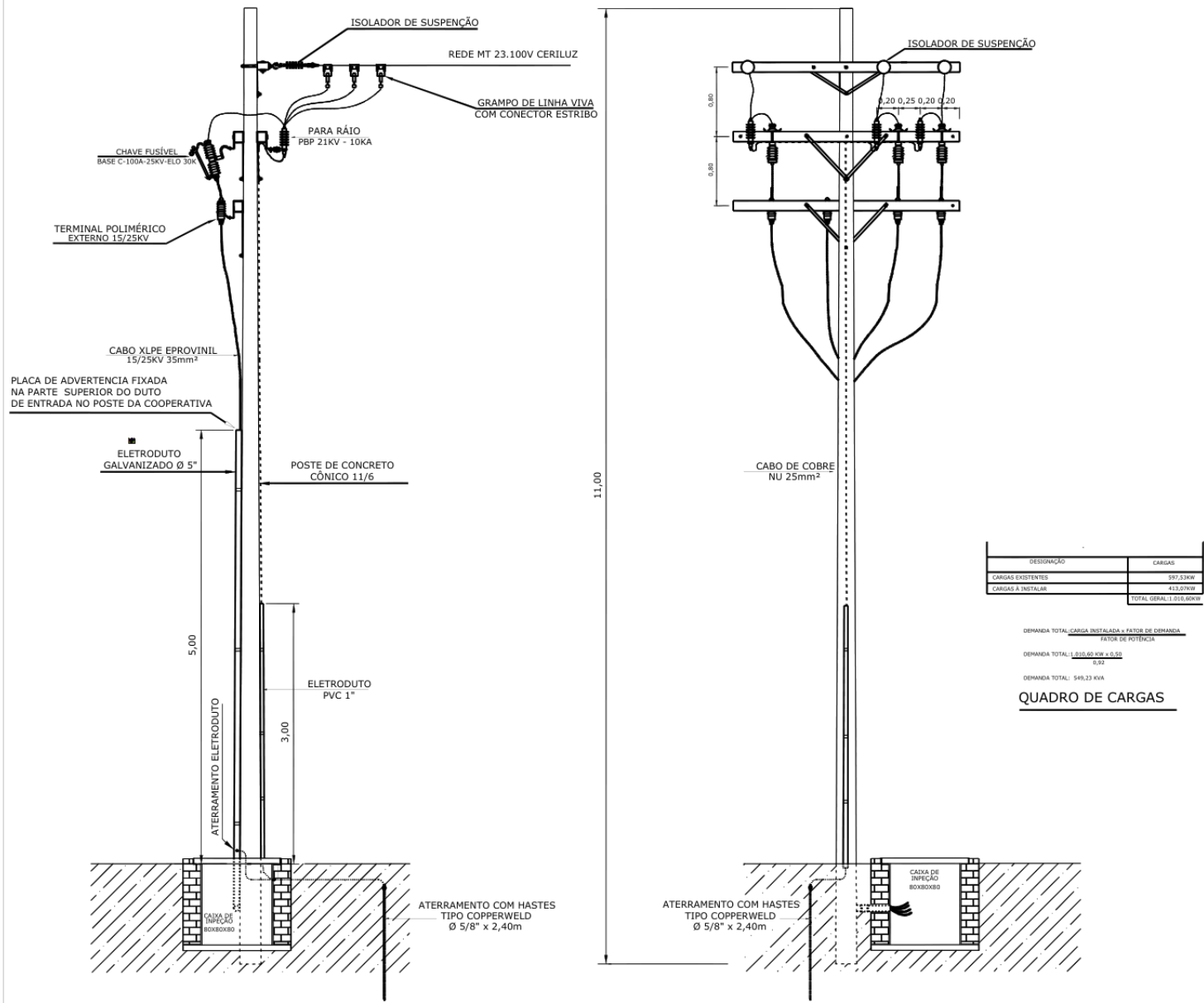
RAMAL DE ENTRADA MT ESCALA - 1:25
