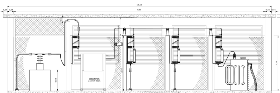
CORTE A - A' ESCALA - 1:25
