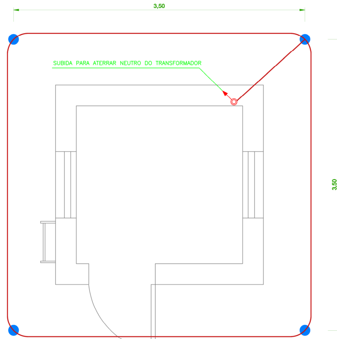
DETALHE DO ATERRAMENTO ESCALA - 1:25
