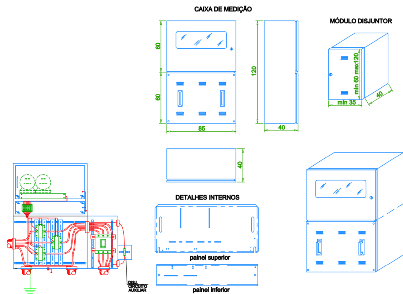
CAIXA DE MEDIÇÃO INDIRETA EM BT ESCALA - 1:25
