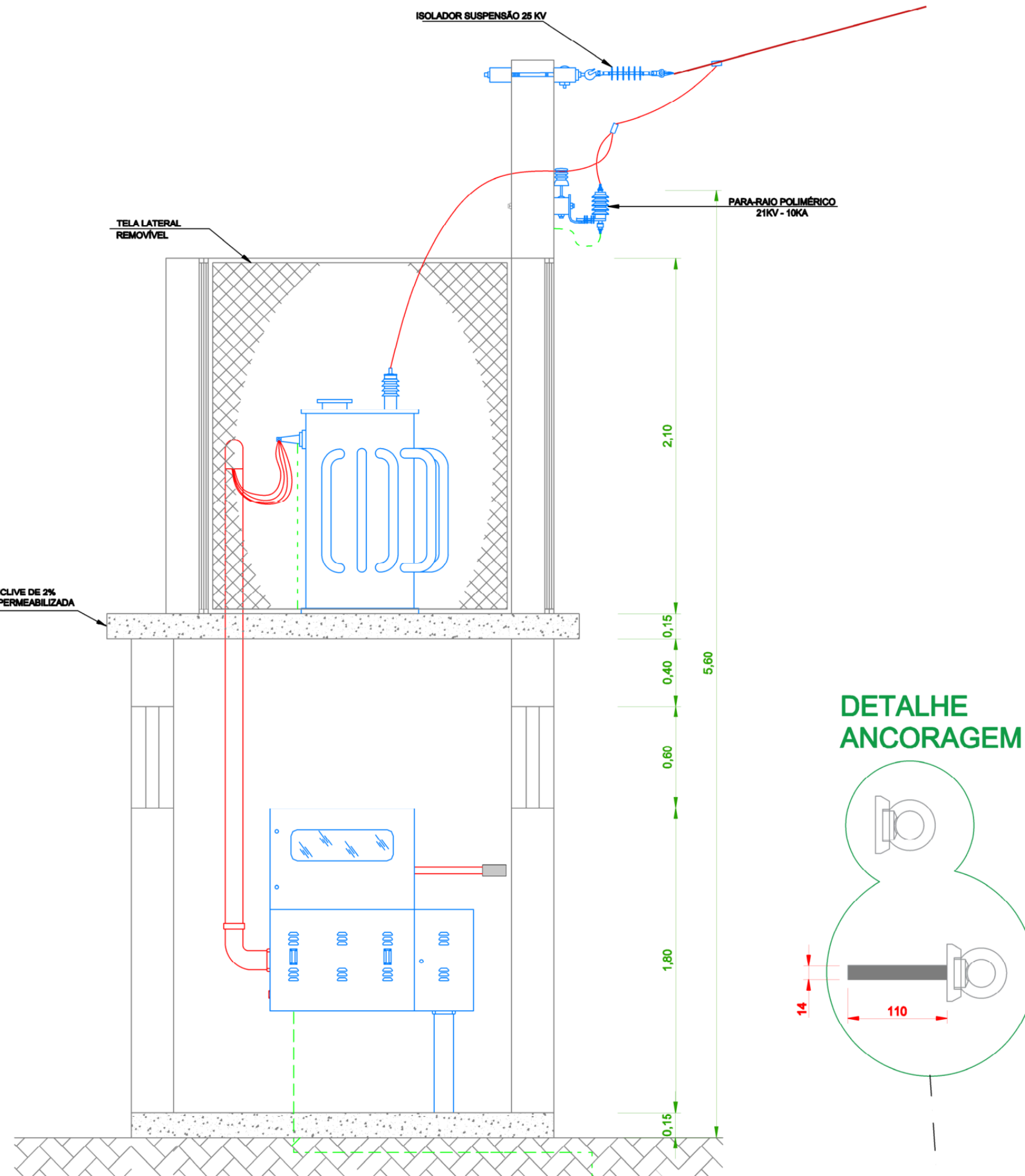
CORTE A - A' ESCALA - 1:25
