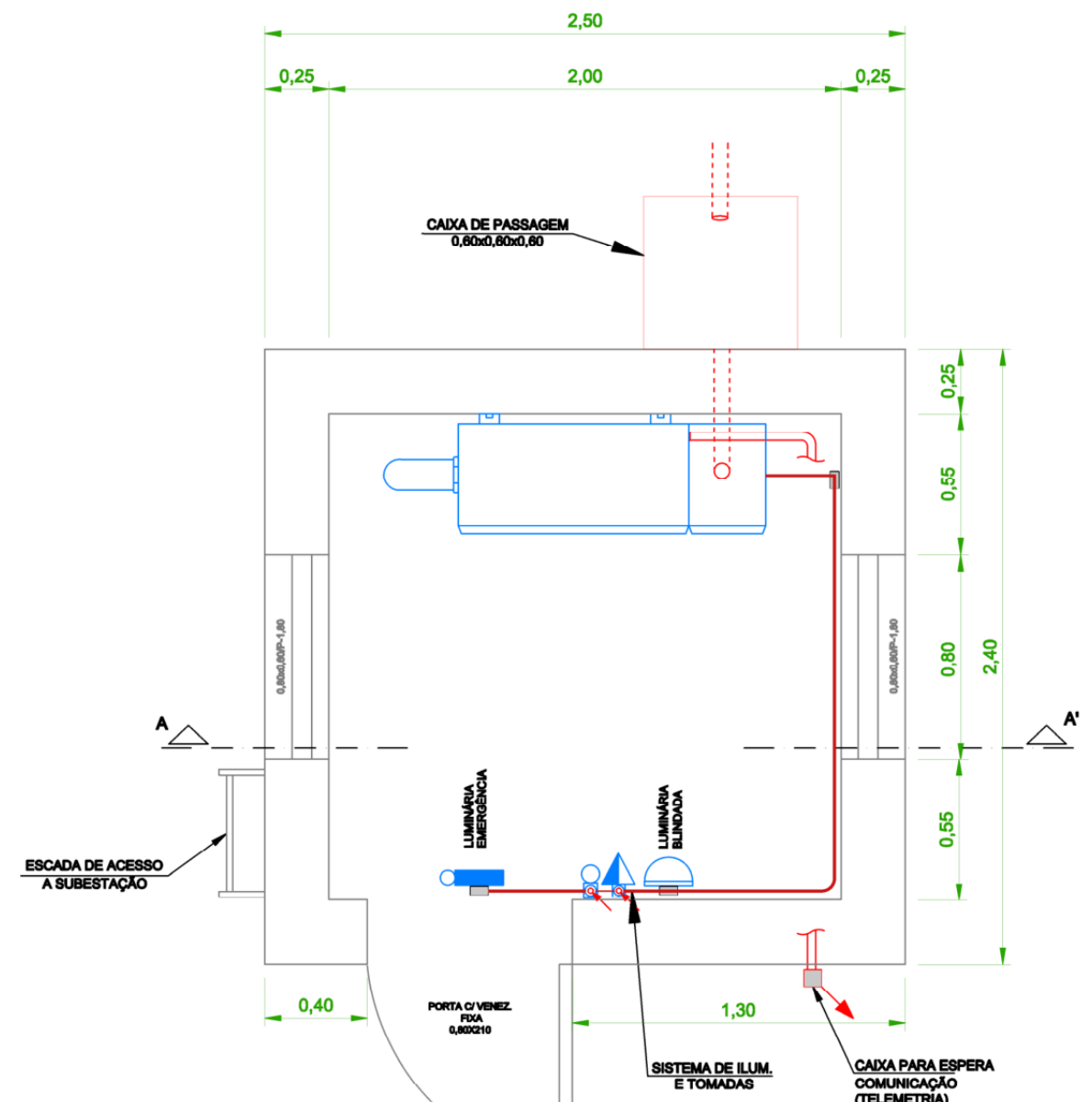
PLANTA BAIXA PAVIMENTO INFERIOR ESCALA - 1:25
