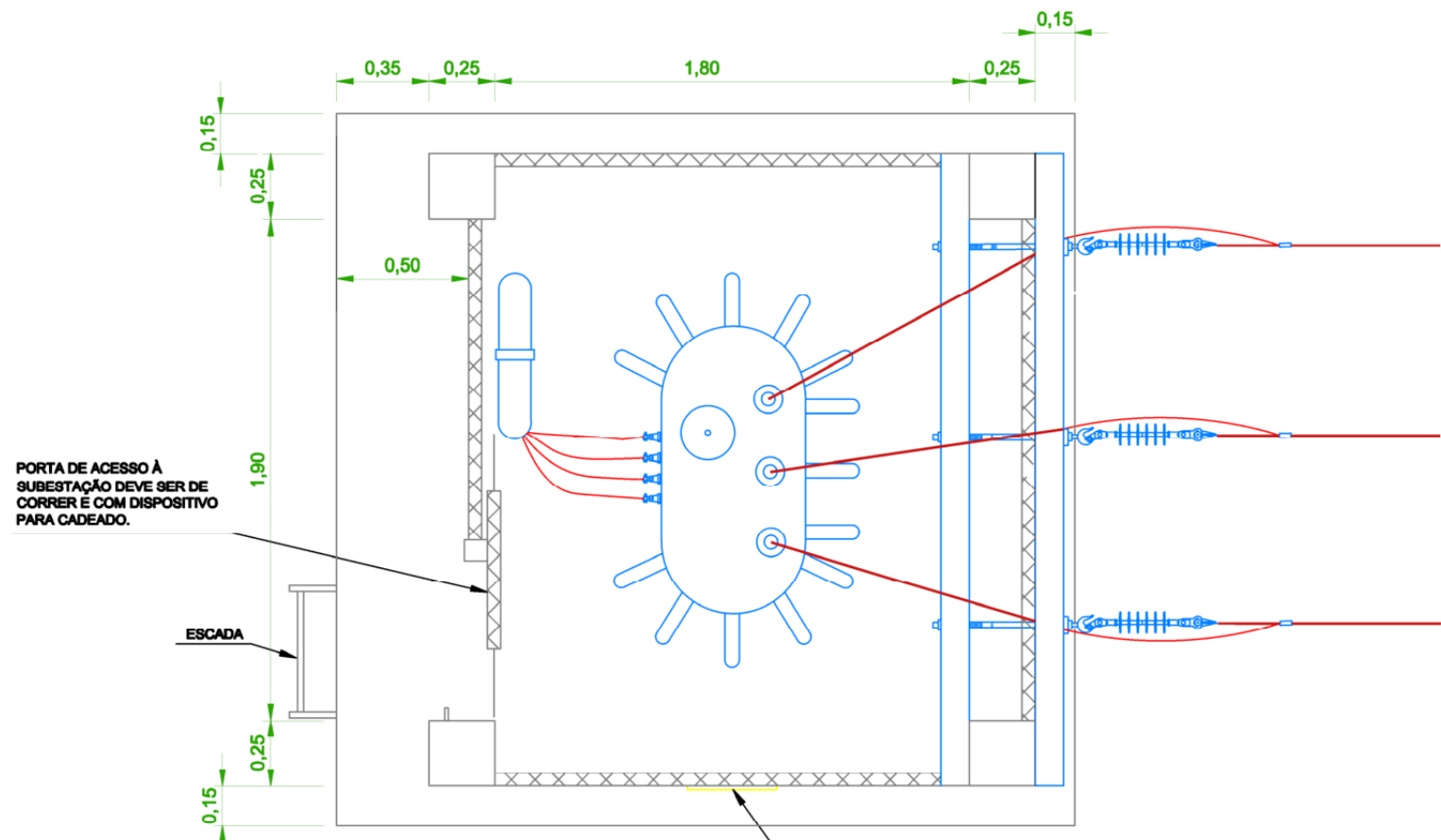
PLANTA BAIXA PAVIMENTO SUPERIOR ESCALA - 1:25
