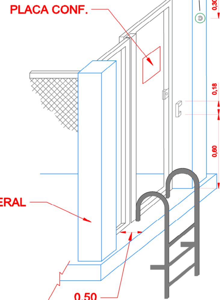
DETALHE DA ESCADA
