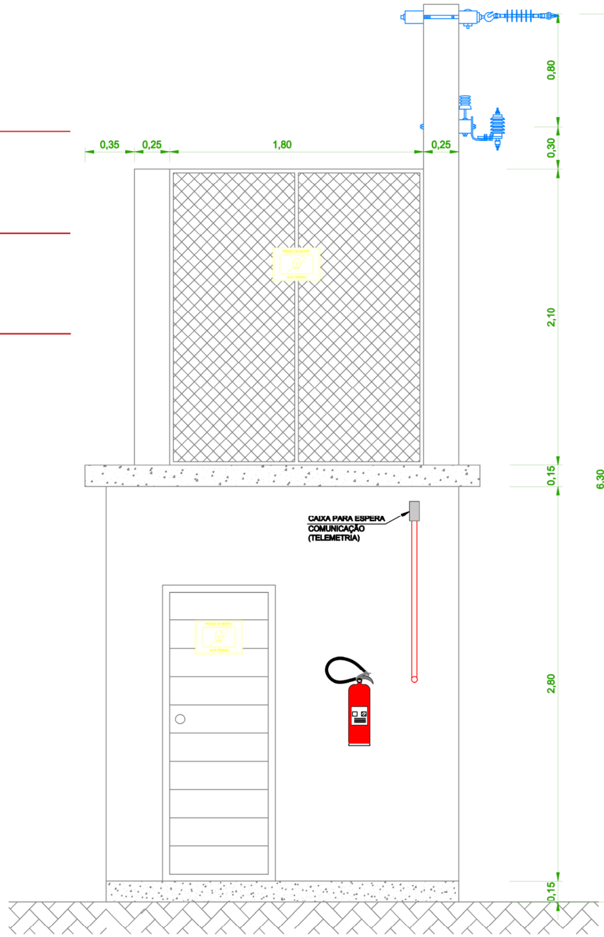
VISTA FRONTAL (FACHADA) ESCALA - 1:25
