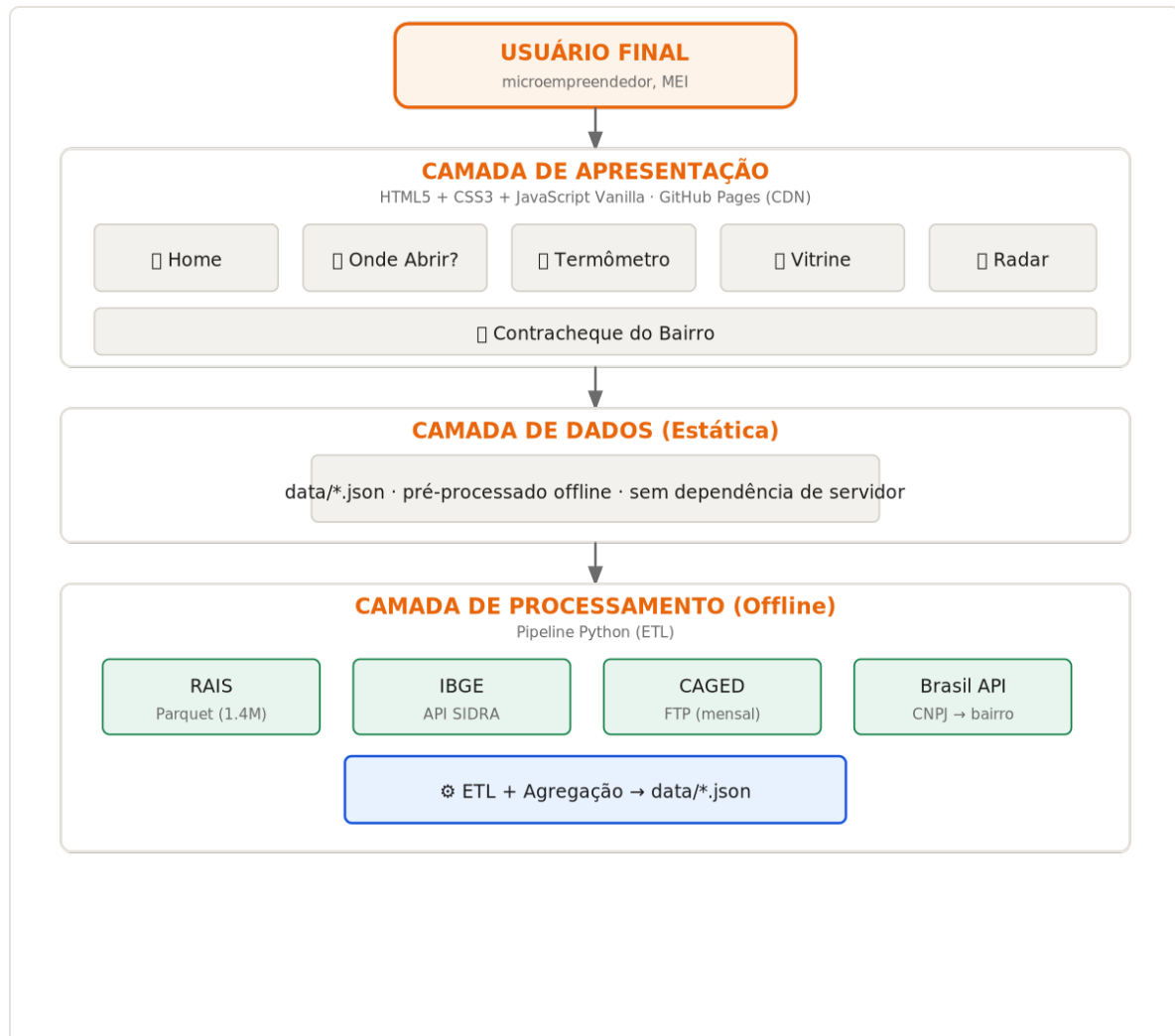
Figura 7: Diagrama detalhado do fluxo — usuário → GitHub Pages CDN → dados JSON estáticos → pipeline ETL offline.
