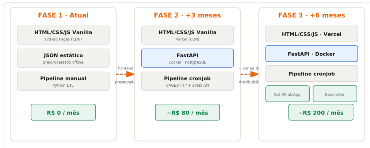
Figura 8: Caminho evolutivo em três fases — do protótipo estático (R$ 0/mês) ao produto multicanal (R$ 200/mês).
