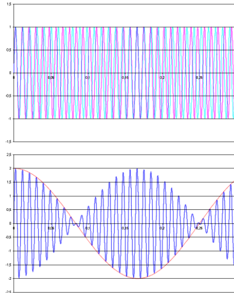
Abbildung 2: Veranschaulichung einer Schwebung. Die beiden oberen Signale mit leicht unterschiedlichen Frequenzen f_1 & f_2 (rot & blau) werden addiert und erzeugen das unten zu sehende resultierende Signal. Dieses besitzt die Frequenz \frac{f_1+f_2}{2} und ändert seine Amplitude mit der Schwebungsfrequenz |f_1 - f_2| . Bildquelle: [2].
