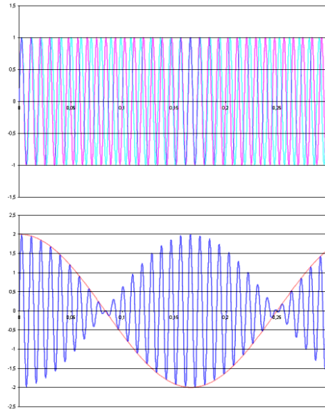
Abbildung 2: Veranschaulichung einer Schwebung. Die beiden Signale mit leicht unterschiedlichen Frequenzen f_1 & f_2 (rot & blau) werden addiert und erzeugen das unten zu sehende resultierende Signal. Dieses besitzt die Frequenz \frac{f_1+f_2}{2} und ändert seine Amplitude mit der Schwebungsfrequenz |f_1 - f_2| . Bildquelle: [1].
