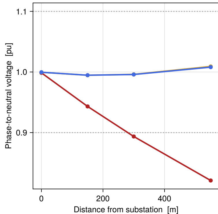
No STATCOM
