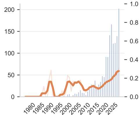
coherence
