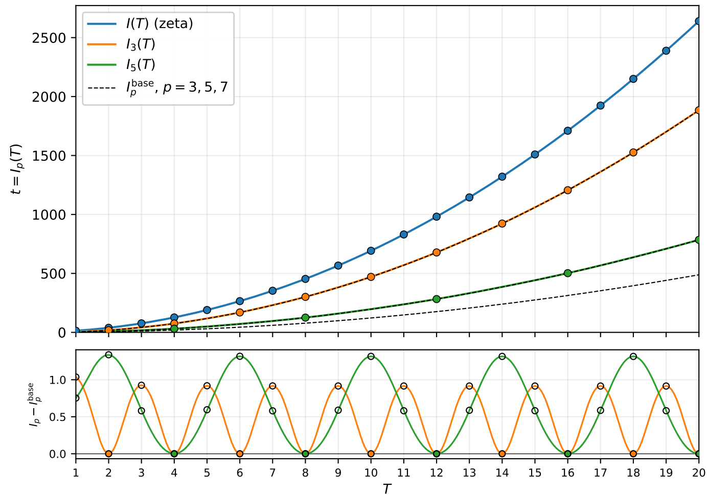
Index maps: l(T) , l_3(T) , l_5(T)
