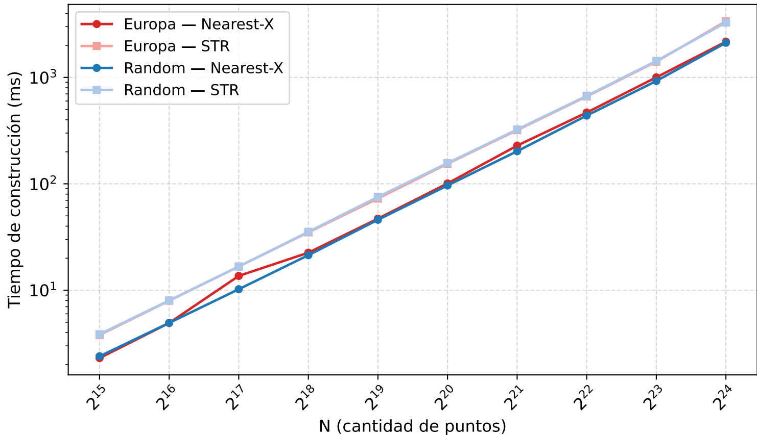
Tiempo de construcción del R-tree vs N
