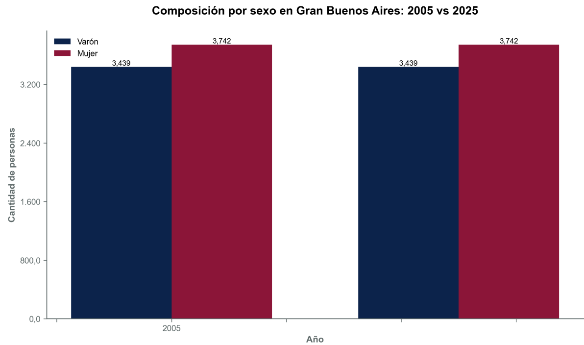
Figura 2: Composición por sexo en Gran Buenos Aires: comparación 2005-2025
