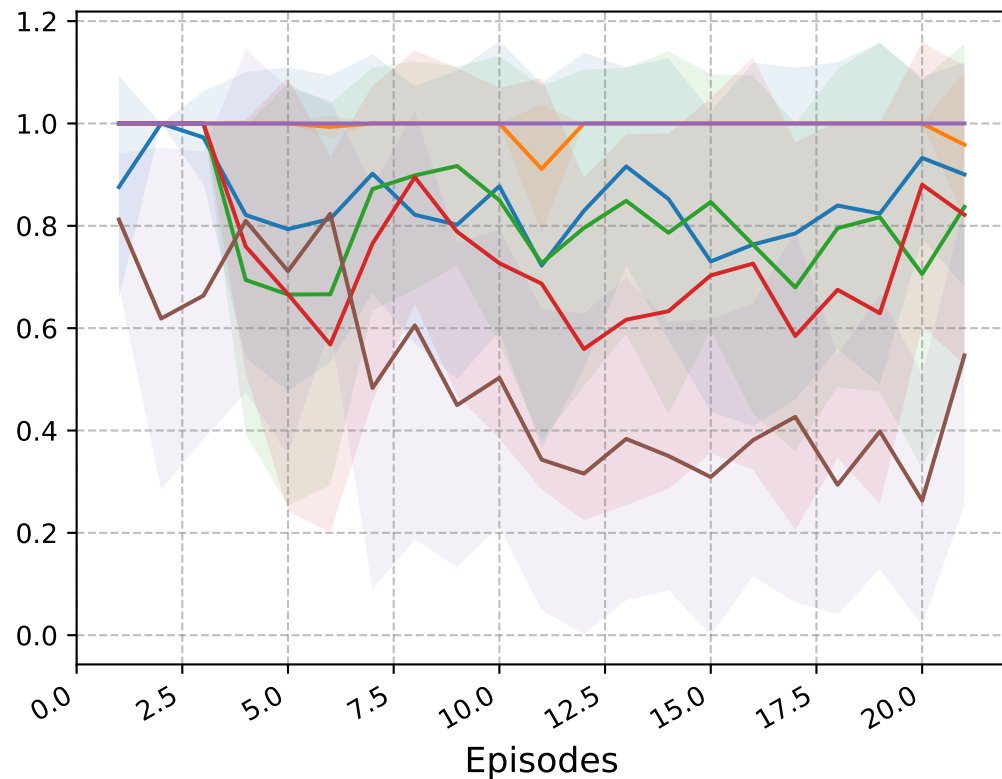
CartPole-v1
