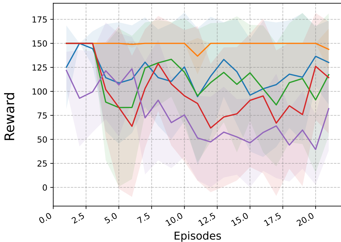
CartPole-v1
