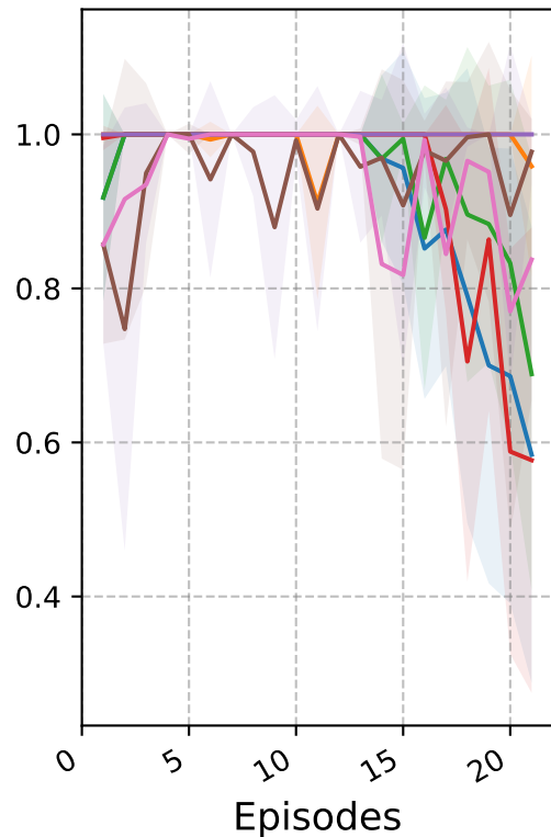
CartPole-v1
