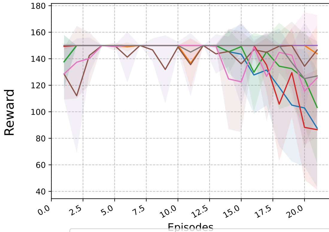
CartPole-v1
