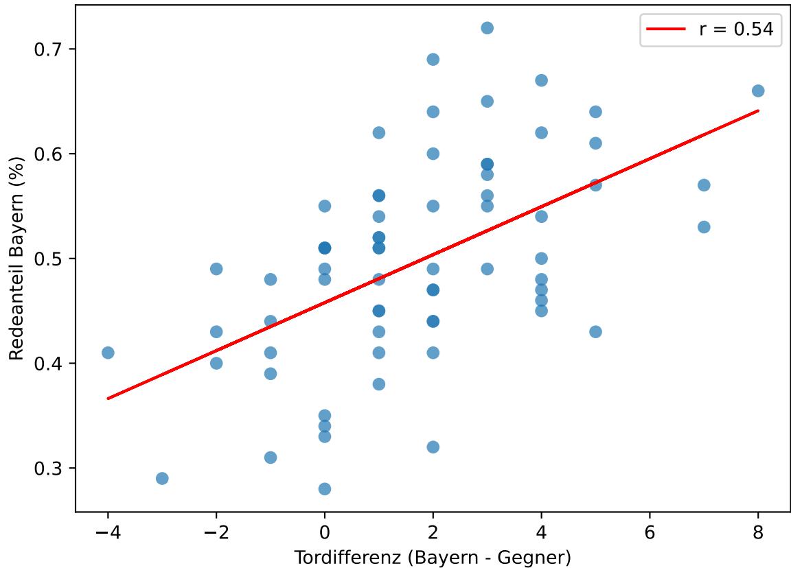
Korrelation: Tordifferenz vs. Redeanteil Bayern
