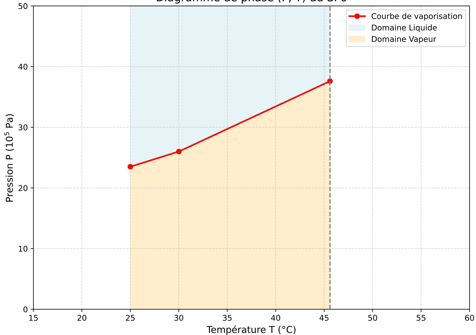
Diagramme de phase (P, T) du SF6
