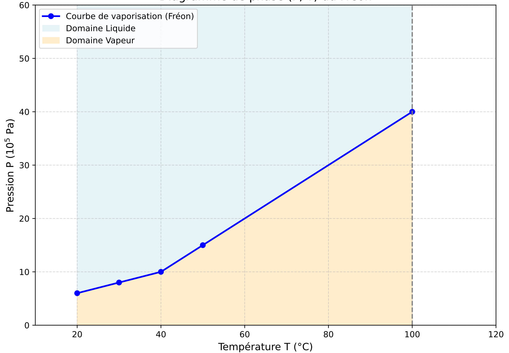
Diagramme de phase (P, T) du Fréon
