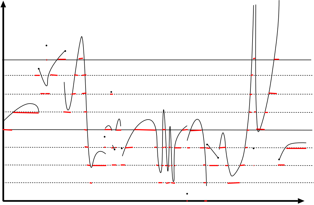
Figure C.7.1: Approximation inférieure d'une fonction f (en noir) par une suite croissante de fonctions étagées.
