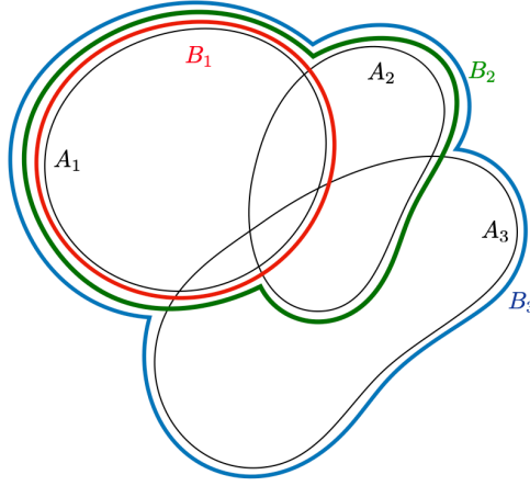
Figure C.2.1: Construction de la suite croissante B_1, B_2, \dots
