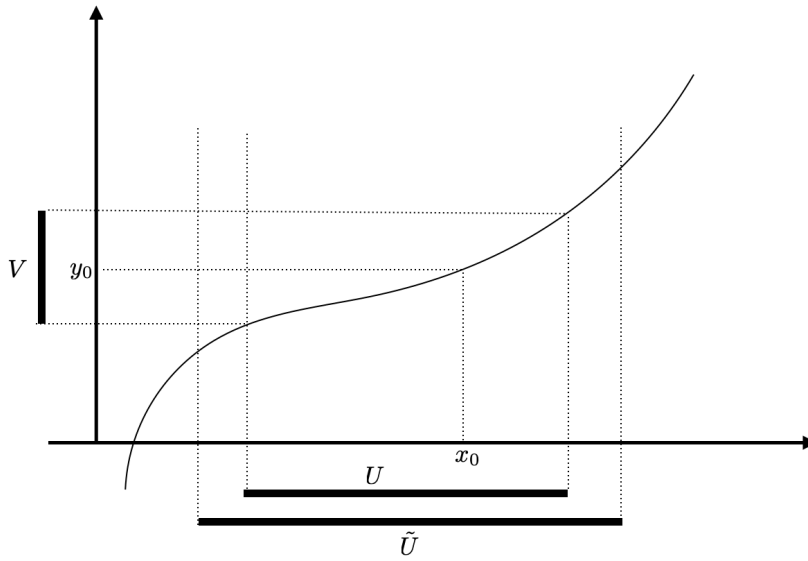
Figure V.2.2: Théorème d'inversion locale
