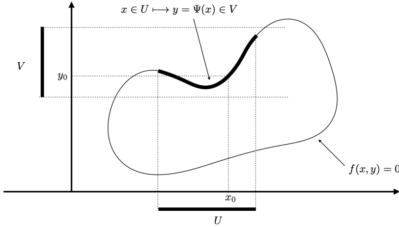
Figure V.2.1: Théorème des fonctions implicites
