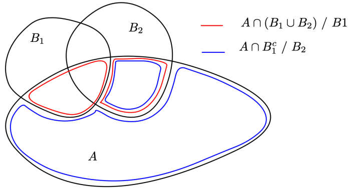
Figure C.4.1: Mesurabilité de B_1 \cup B_2 . La notation C / D de la légende indique que l'on écrit C comme l'union de C \cap D et de C \cap D^c , où D est un ensemble mesurable.
