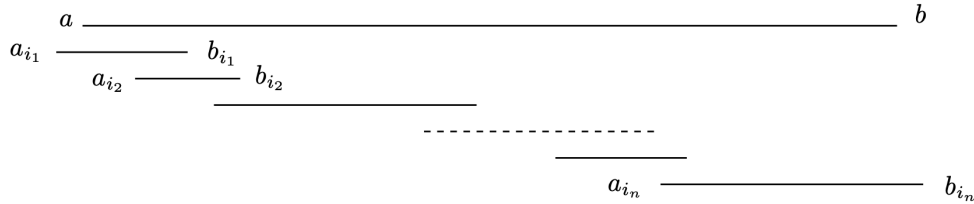
Figure C.4.2: Recouvrement d'un intervalle
