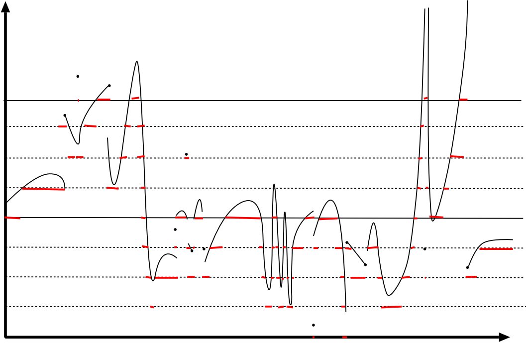
Figure C.7.1: Approximation inférieure d'une fonction f (en noir) par une suite croissante de fonctions étagées.
