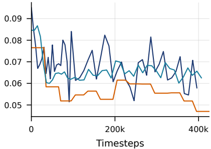
WFG6_3
